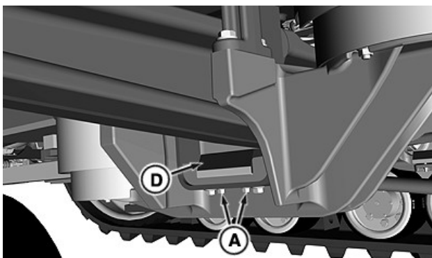
A—Mutter (2 st.) D—Höger undre stötdämparstopp
