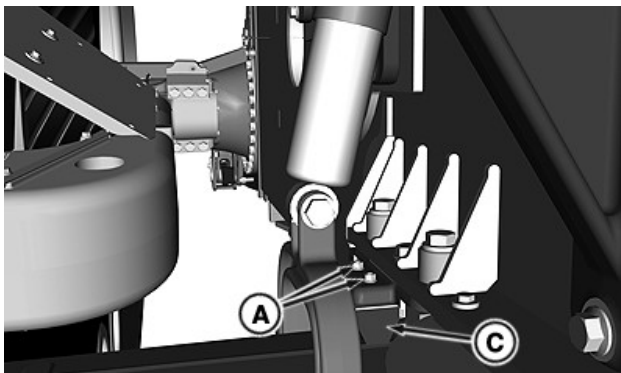
A—Mutter (2 st.) C—Höger övre stötdämparstopp
