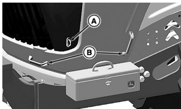
Huvlossning och huvhandtag
