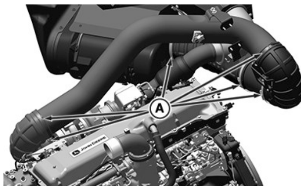
Enkelturbomotor
