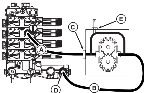
Sprutpump—Utan lyft
