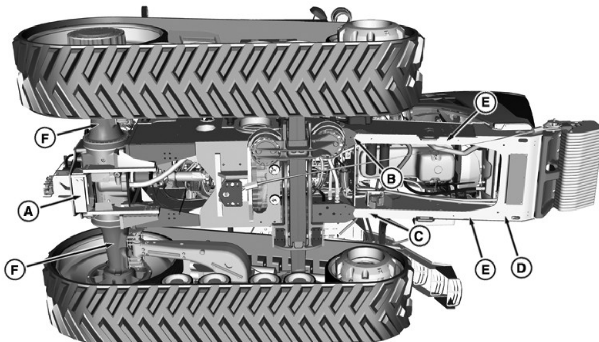
Lyftpunkter på undersida
