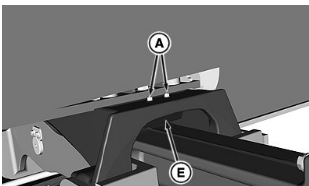
A—Mutter (2 st.) E—Vänster övre stötdämparstopp
