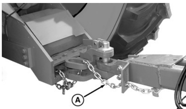
Vanlig dragbom
