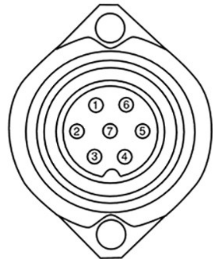
Schemat wylotowy ISO 11786
