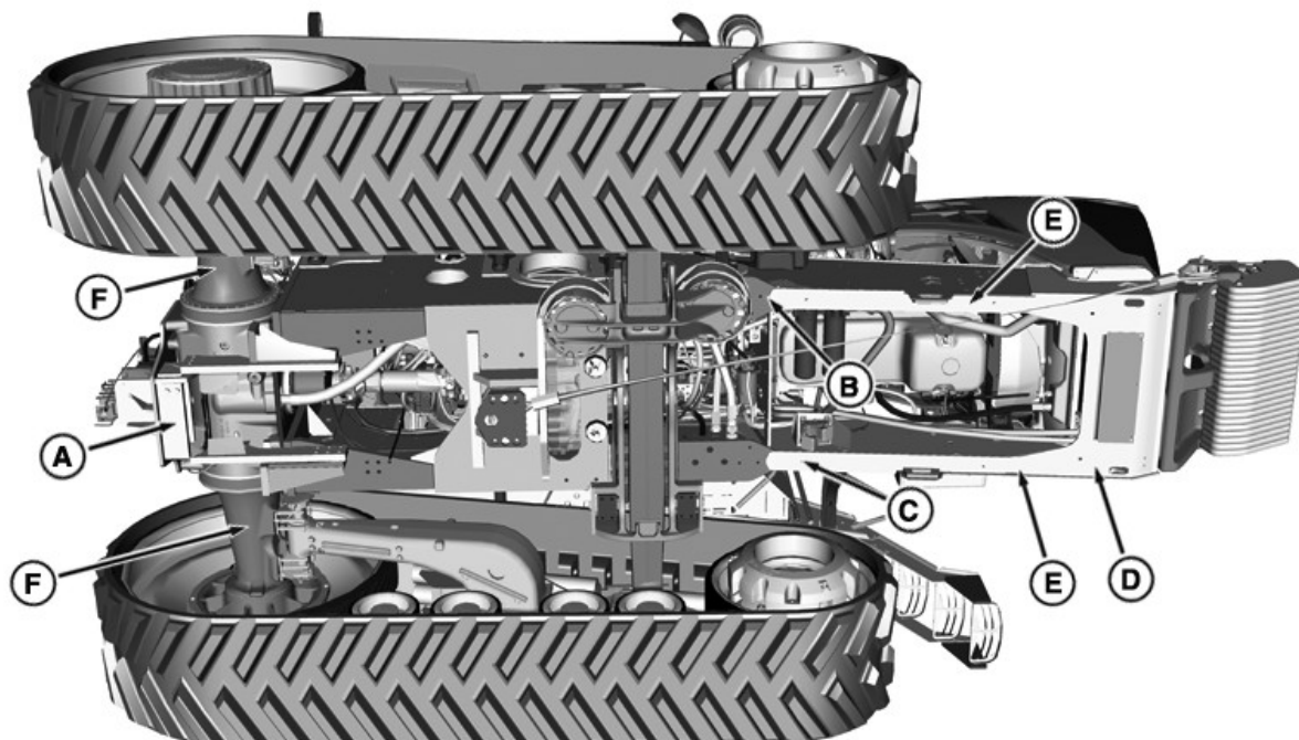
Punkty podnoszenia na spodzie
