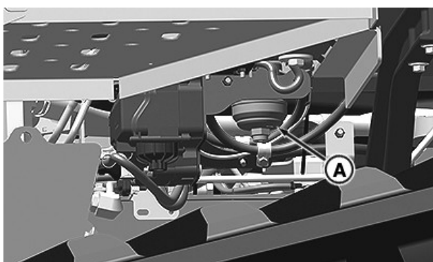
RXA0185240—UN—26AUG21 Filtr liniowy DEF (A) znajduje się pod lewymi stopniami.
