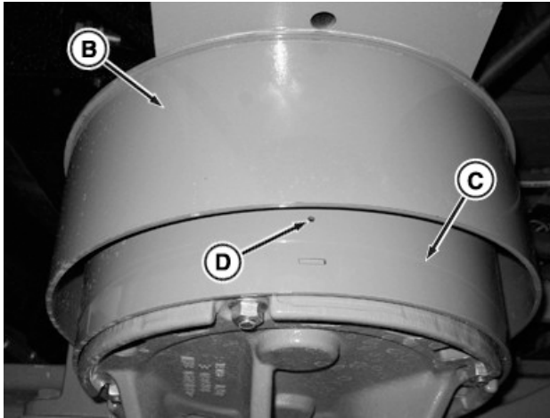
Pneumatyczna amortyzacja
