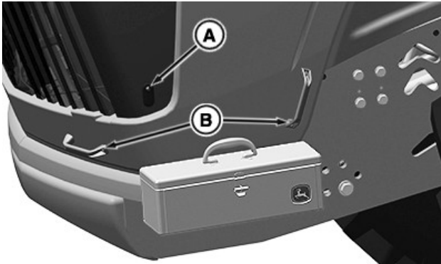
RXA0180141—UN—15OCT20 Przycisk zwalniania i uchwyty maski
