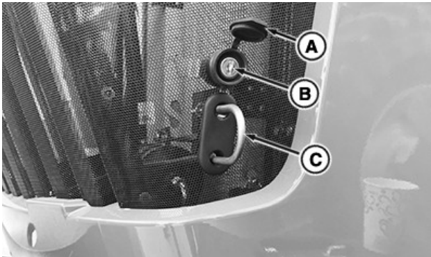
RXA0163079—UN—27APR18 Pokrywa, blokada i zatrask maski
