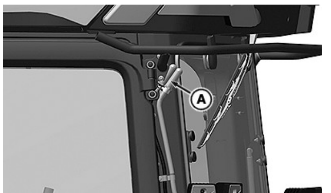
RXA0180428—UN—11NOV20 Filtr odpowietrznika zbiornika DEF (A) znajduje się w górnej części lewego tylnego narożnika kabiny.
