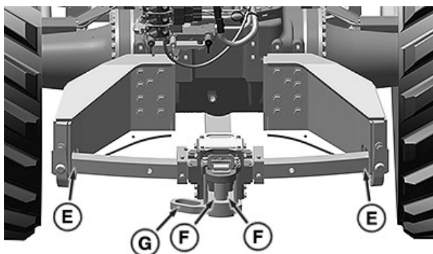
С широко завъртащ се теглителен прът
