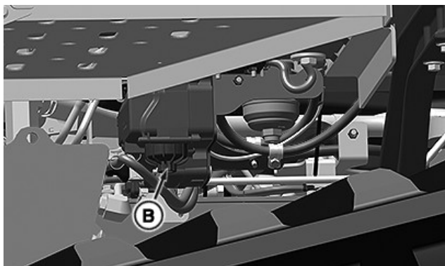
RXA0185241—UN—26AUG21 Филтърът на модула за дозиране на DEF (В) се намира под левите стъпки.
