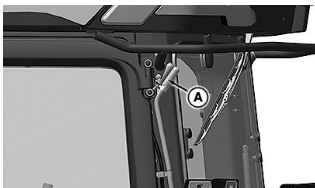
Вентилационният филтър на резервоара DEF (A) е близо до горната част на задния ляв ъгъл на кабината.
