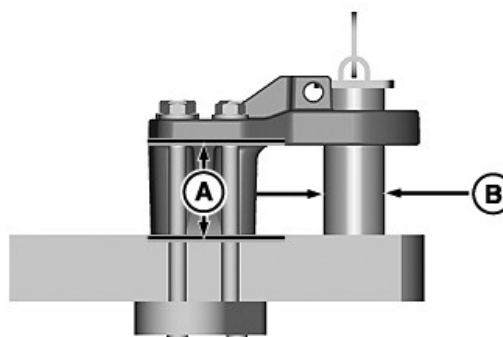
Размери на звеното на навесната система
