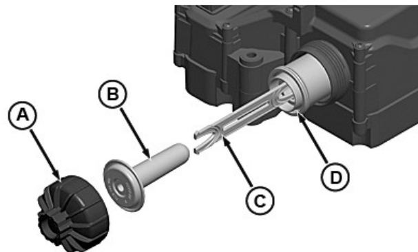
Filter dávkovacej jednotky DEF
