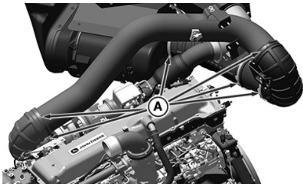
Jednostupňový turbo motor
