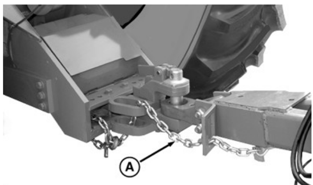
RXA0058318—UN—06NOV01 Normálne tiahlo
