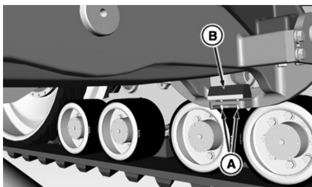
A—Matica (2 ks) B—Ľavá spodná tlmiaca zarážka
