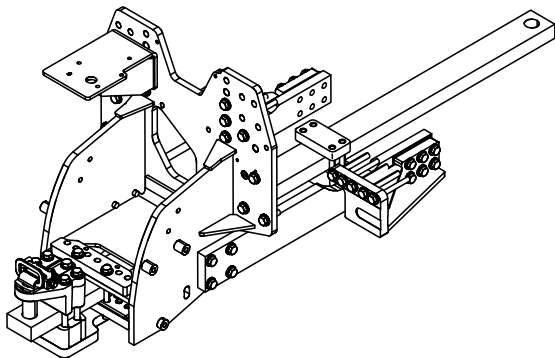
RXA0074740—UN—03MAY04 Halterung für Zugpendel in verstärkter Ausführung, Kapazität 4990 kg (11000 lb)
