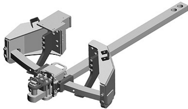
RXA0098007—UN—06MAY08 Halterung für Zugpendel mit großem Schwenkbereich mit Montagesatz für Schwerlast-Halterung, Kapazität 5440 kg (12000 lb)
