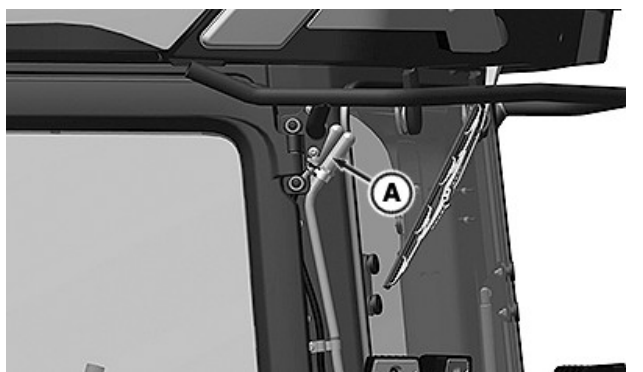
RXA0180428—UN—11NOV20 Der Entlüftungsfilter des DEF-Tanks (A) befindet sich in der Nähe der oberen linken Ecke der Kabine.
