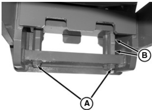
Einrichtung der Halterung für das größere Schürfkübel-Zugpendel
