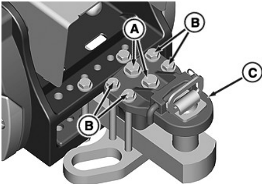
RXA0141899—UN—05JUN14 Zugpendel in verstärkter Ausführung
