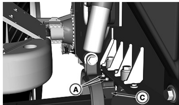
Labais augšējais bufera atduris
