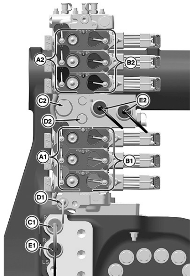
A1—Izbīdīšanas savienotājs (primārais hidrauliskais sūknis) (3 gab.)
