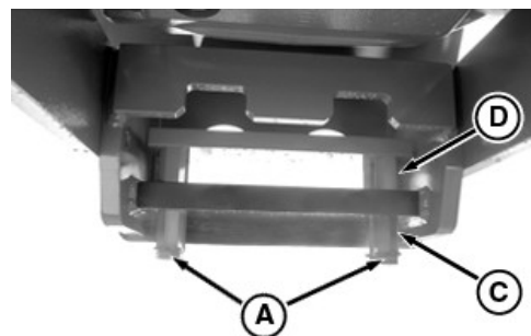
Īsā skrēpera jūgstieņa balsta uzstādīšana
