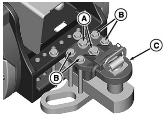
Lielas noslodzes jūgstienis
