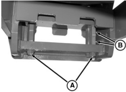
Garāka skrēpera jūgstieņa balsta uzstādīšana
