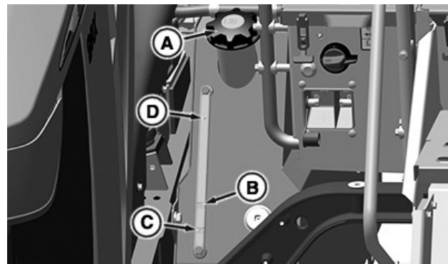
Visor de Nível de Óleo Hidráulico/Transmissão
