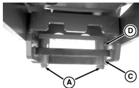
Inställning för mindre fäste till avskrapardragbom
