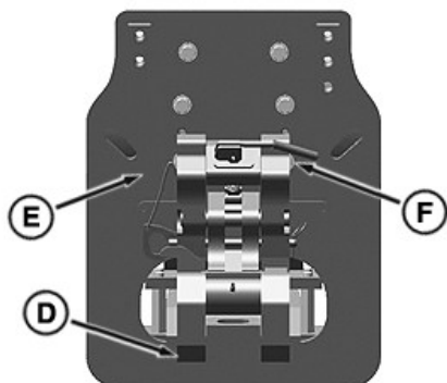
Snabbkoppling till dragbom
