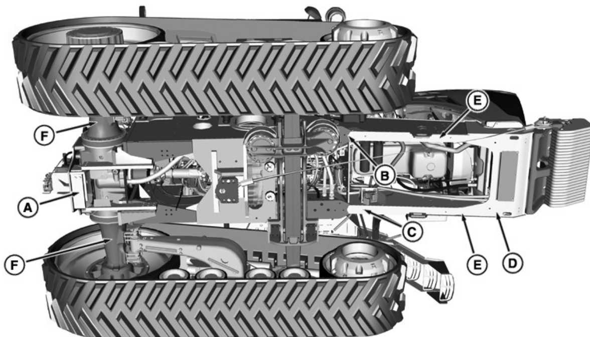
Undersida, lyftpunkter
