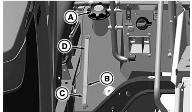
Siktglas för transmissions-/hydraulolja
