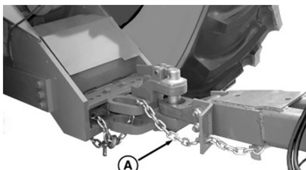
Brett svängbar dragbom
