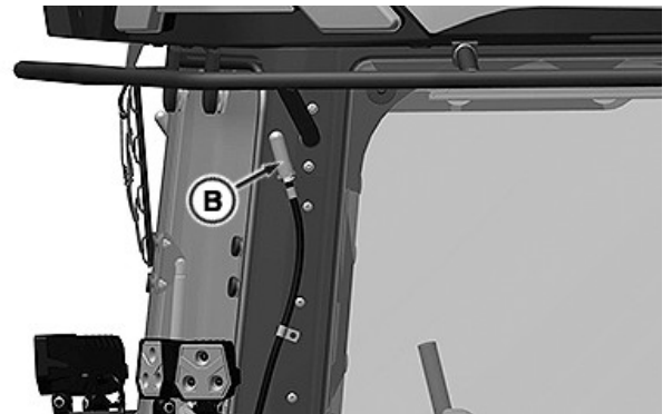
Odvdzušňovací filter palivovej nádrže (B)-pravý zadný rohový stĺpik kabíny
