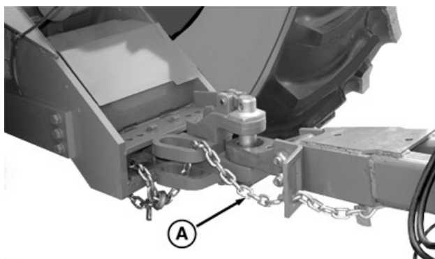
Normálne tiahlo
