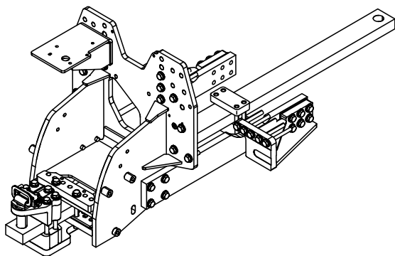
RXA0074740—UN—03MAY04 Wspornik wzmacniający do zaczepu rolniczego, udźwig 4990 kg (11000 lb.)
