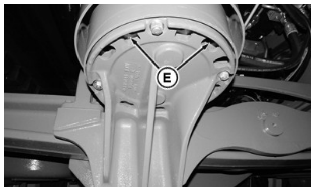
Poduszka powietrzna przedniego wahacza
