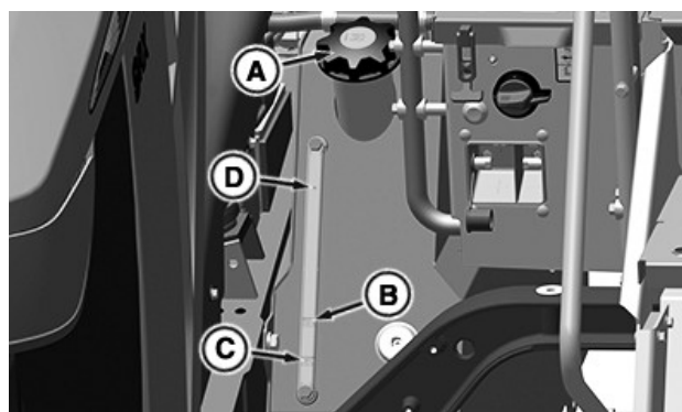
Okienko wskaźnika poziomu oleju przekładniowego/hydraulicznego
