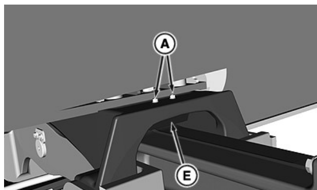
A—Nakrętka (2 szt.) E—Lewy górny ogranicznik zderzaka
