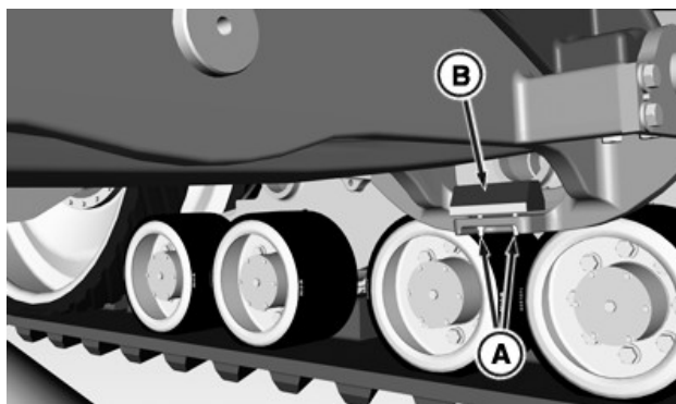
A—Nakrętka (2 szt.) B—Lewy dolny ogranicznik zderzaka
