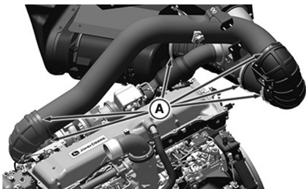
Silnik z jednostopniową turbosprężarką
