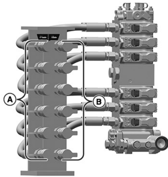
A—Port wysuwania (6 szt.) B—Port cofania (6 szt.)
