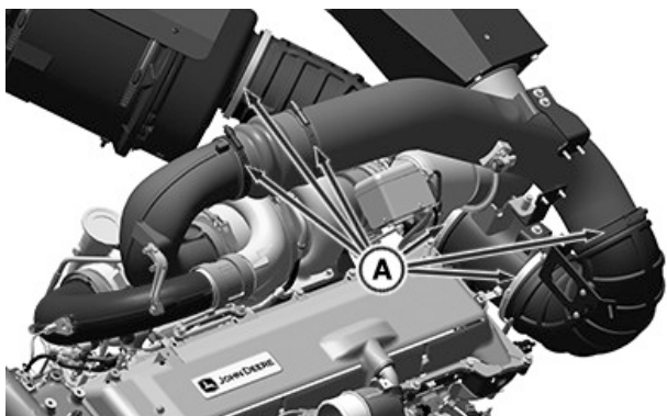
Silnik z dwustopniową turbosprężarką
