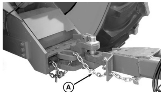
RXA0058318—UN—06NOV01 Standardowy zaczepek rolniczy
