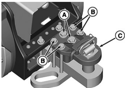
RXA0141899—UN—05JUN14 Zaczep rolniczy wzmocniony
