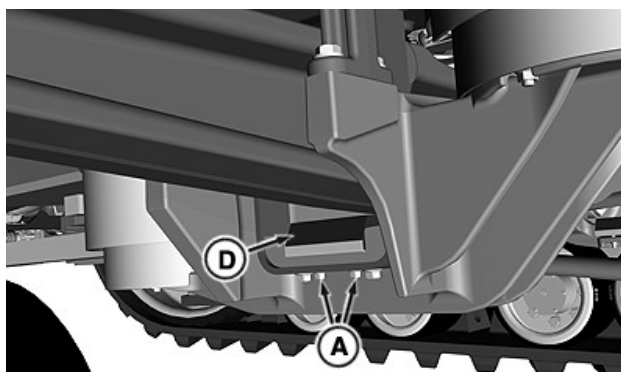
A—Nakrętka (2 szt.) D—Prawy dolny ogranicznik zderzaka
