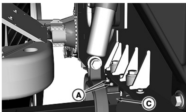
A—Nakrętka (2 szt.) C—Prawy górny ogranicznik zderzaka
