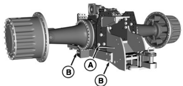
Wspornik sztywnego zaczepu rolniczego
