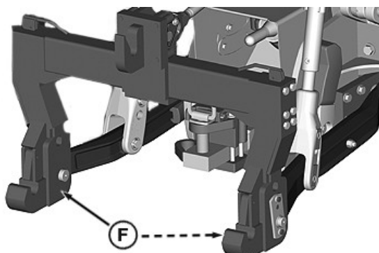
Attelage rapide illustré dans la configuration de catégorie 4N
