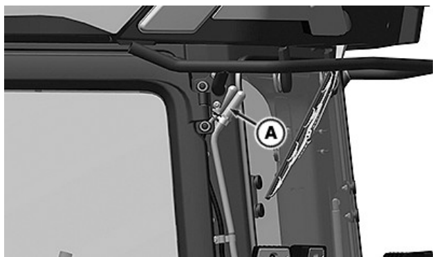
RXA0180428—UN—11NOV20 Le filtre de l'orifice de dégazage du réservoir d'urée DEF (A) se trouve près du coin supérieur arrière gauche de la cabine.
