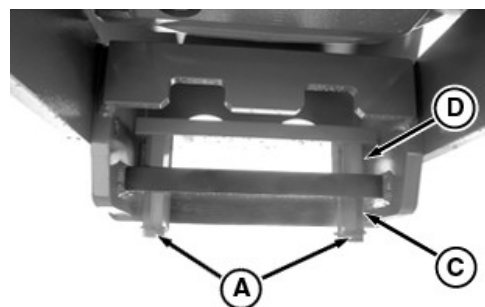
Налаштування опори для меншого тягово-зчіпного пристрою грейдера
