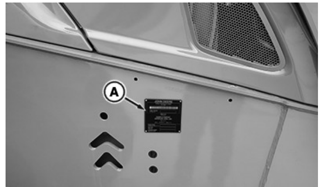
Табличка з ідентифікаційним номером виробу (A) розташована на правому боці рами трактора
