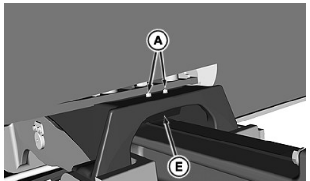
А—Гайка (2 шт.) Е—Лівий верхній буферний упор
