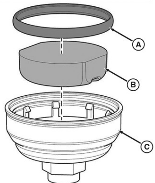
Компоненти корпусу фільтра
