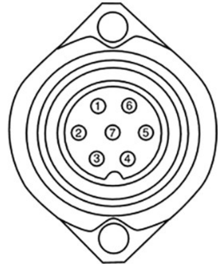
РХА0169832—UN—05AUG19 Схема виводу ISO 11786
