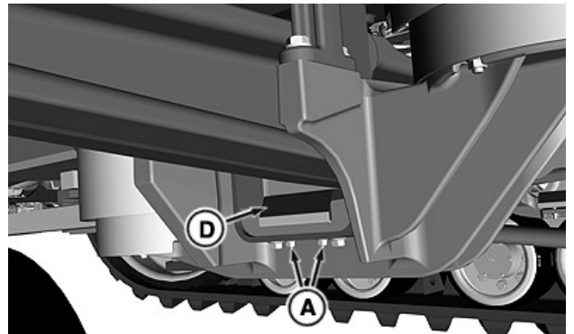
А—Гайка (2 шт.) D—Правий нижній буферний упор
