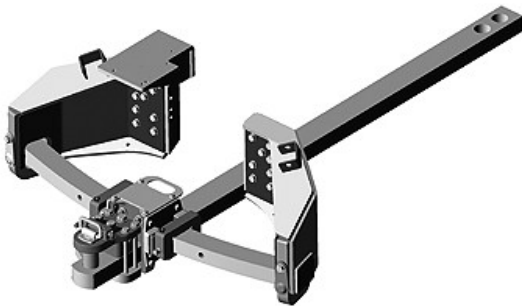
Опора маятникового тягово-зчіпного пристрою з широким кутом повороту, вантажність 4580 кг (10100 фунтів)
