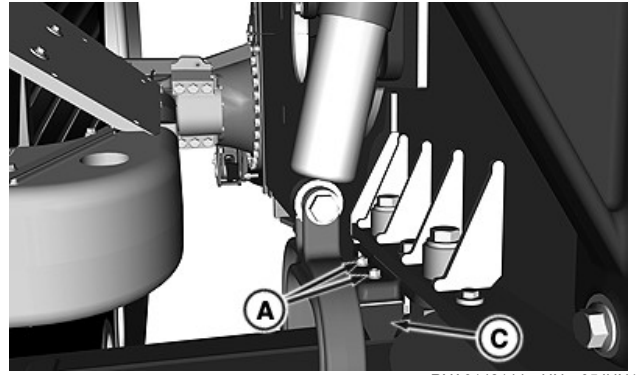
А—Гайка (2 шт.) С—Правий верхній буферний упор
