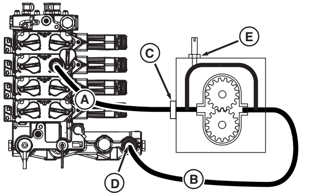
Спринклерний насос (без зчіпки)
