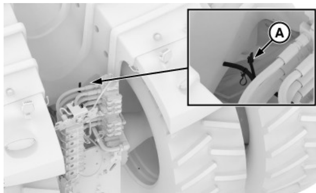
Роз'єм датчика тягового зусилля
