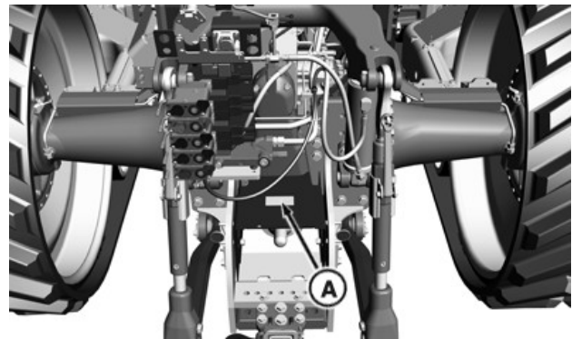
A—Табличка ВОМ (задняя часть трактора на щитке ВОМ)
