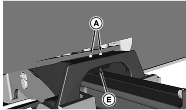
A—Tuerca (se usan dos) E—Tope del amortiguador superior izquierdo
