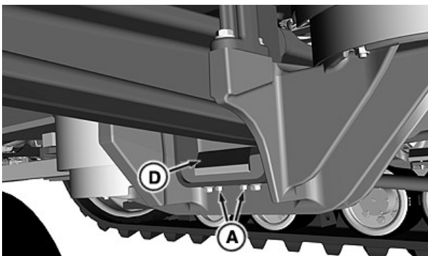
A—Tuerca (se usan dos) D—Tope del amortiguador inferior derecho
