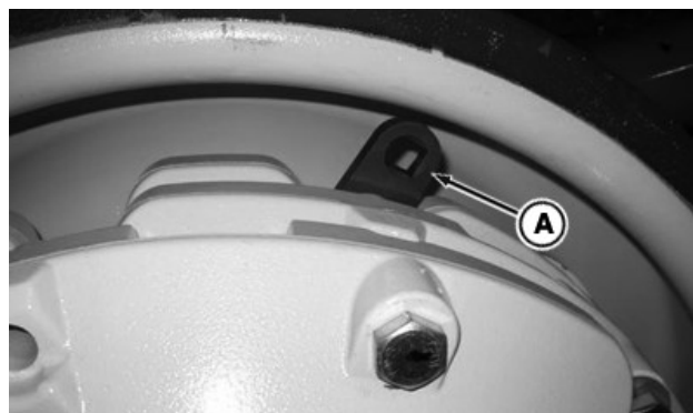
RXA0100328—UN—03FEB09 Llave de sujeción de contrapesos de rueda JDG10958
