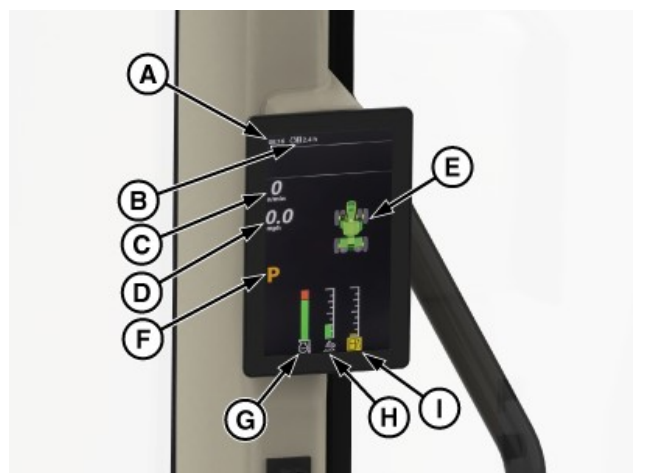
RX1361839—UN—27MAR24 Pantalla del poste derecho
