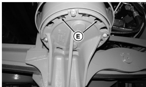
Cojín de aire del balancín frontal
