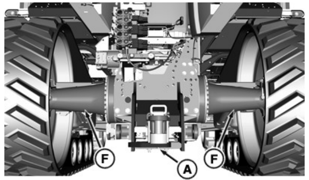
Punto de elevación trasero
