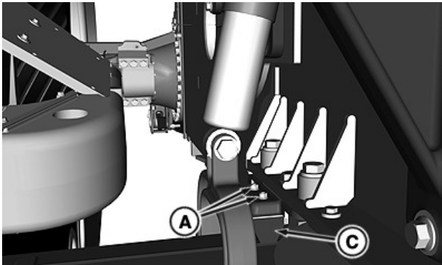
A—Tuerca (se usan dos) C—Tope del amortiguador superior derecho
