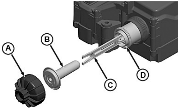
RG22534—UN—21MAR13 Filtro de la unidad de dosificación de DEF
