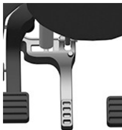
Педаль наклона с запоминанием положения
