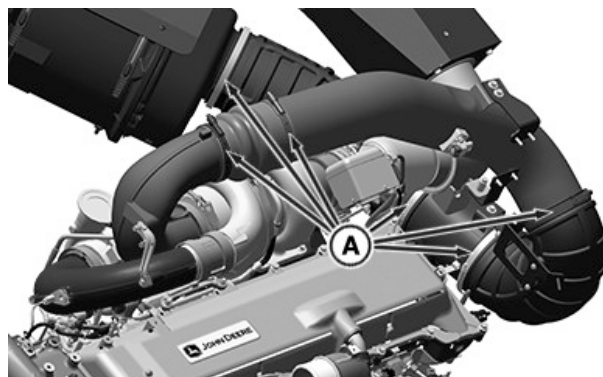
Двигатель с двумя турбокомпрессорами
