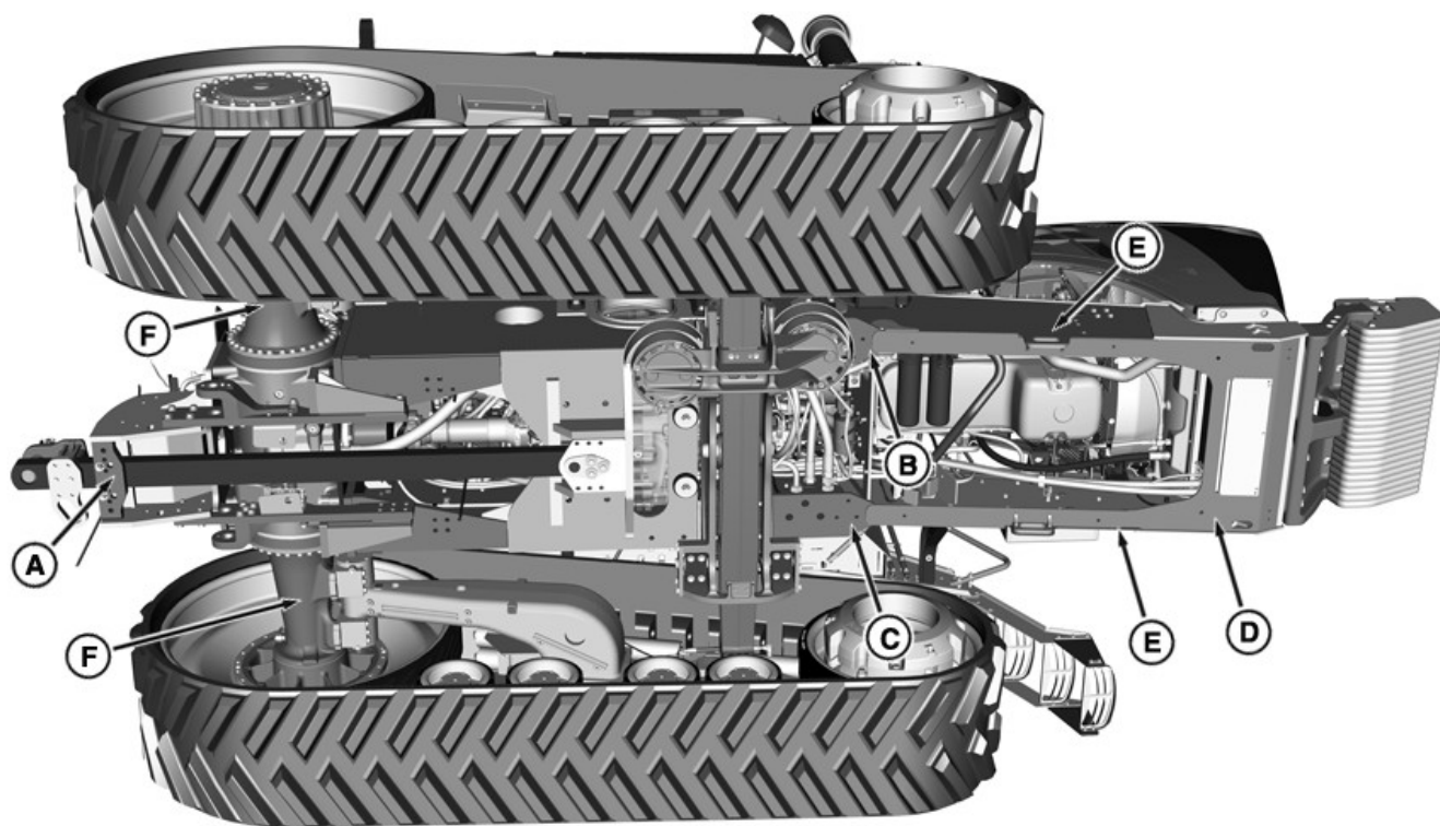
Вид снизу, поддомкратные площадки
