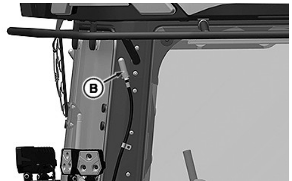
Фильтр вентиляции топливного бака (В) — правая задняя угловая стойка кабины
