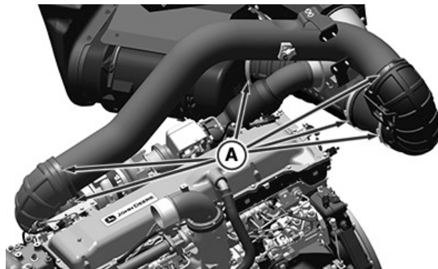
Двигатель с одним турбокомпрессором
