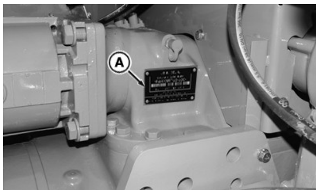
RXA0142510—UN—12JUN14 Табличка с серийным номером моста (А) расположена на картере заднего моста
