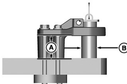
Dimensiunile articulației de cârlig
