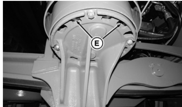
Burduful de aer al balansierului din față
