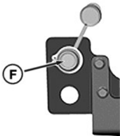
Identificarea și localizarea componentelor [Ag] — sisteme hidraulice cu debit mare: (F) Cupla băii—Drenarea carterului motorului
