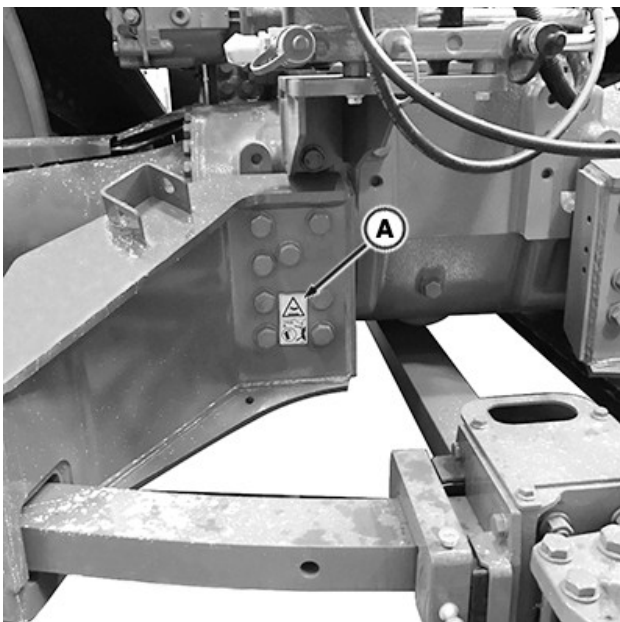
A—Nalepka "Gorąca powierzchnia"
