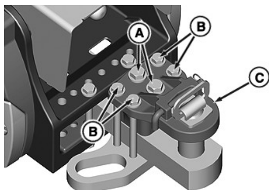
Wzmocniony zaczep rolniczy
