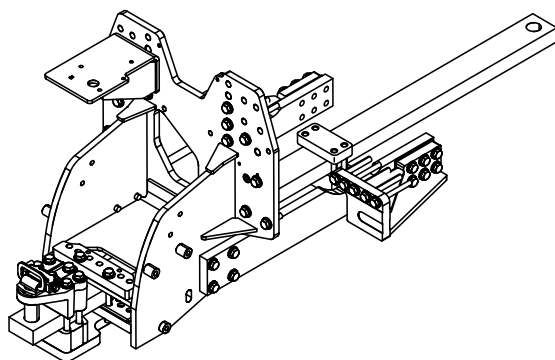
Wspornik wzmacniający do zaczepu rolniczego, udźwig 4990 kg (11000 lb.)
