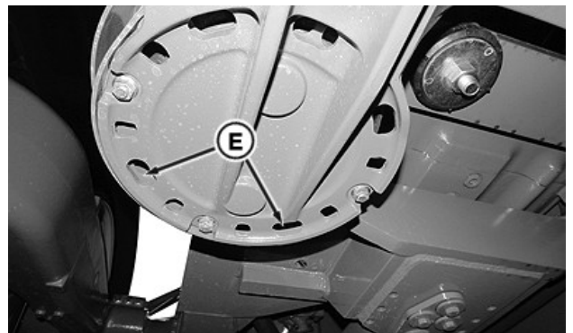
Poduszka powietrzna tylnego wahacza
