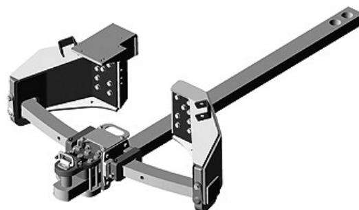
Wspornik zaczepu rolniczego o szerokim promieniu wychylenia, udźwig 4580 kg (10100 lb.)
