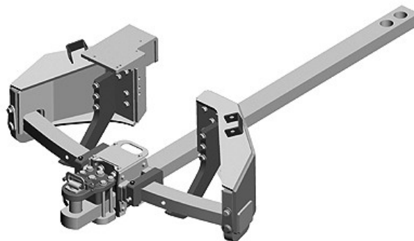
Wspornik zaczepu rolniczego o szerokim promieniu wychylenia z zestawem wspornika wzmacniającego, udźwig 5440 kg (12000 lb.)
