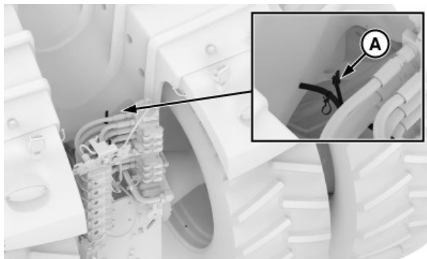
Veojõuanduri juhtmekimbu ühendus
