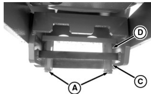
Skreepri väiksema haakeraua kanduri häälestus
