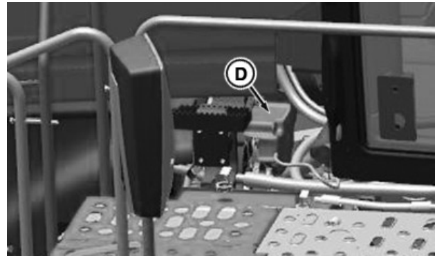
Peakaitsete paneel (D) asub kapoti alumise toe vasakul tagaküljel.
