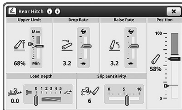
Tagumise rippüsteemi näide
