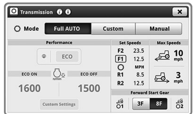
Mjenjač
