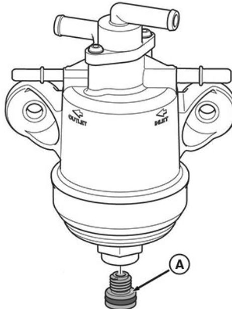
RG30728—UN—08AUG18 Vidange de l'urée DEF
