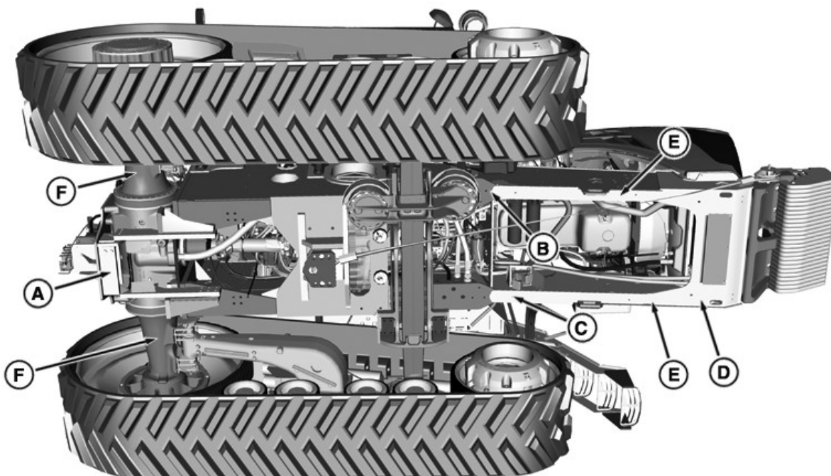
Долна страна, точки за вдигане
