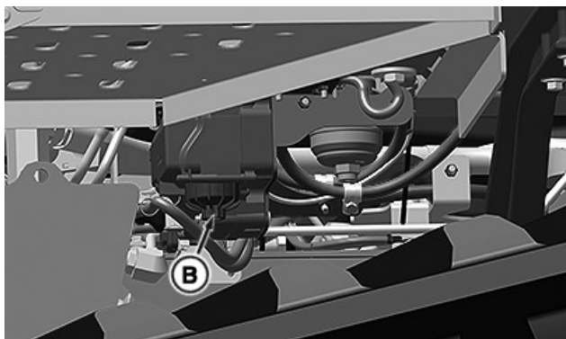
Филтърът на модула за дозиране на DEF (B) се намира под левите стъпалки.
