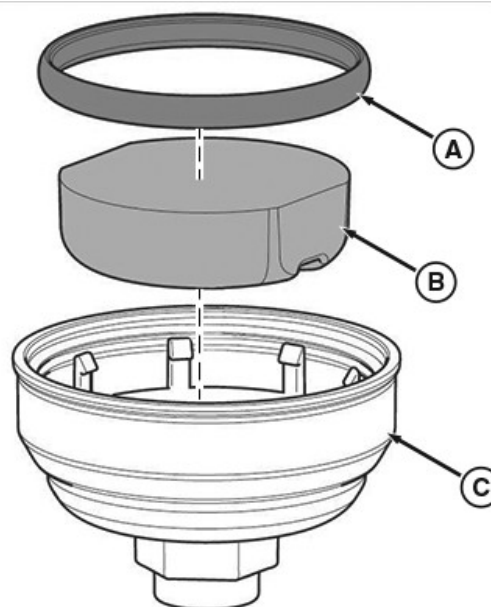
Компоненти на корпуса на филтъра
