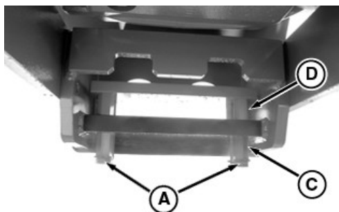
Настройка на опората на по-малкия теглич на скрепера
