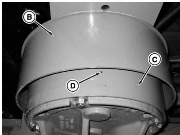
Въздушно окачване
