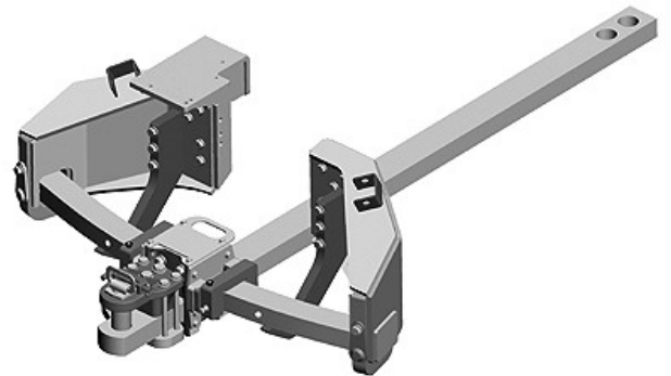
RXA0098007—UN—06MAY08 Support de barre d'attelage à grand débattement avec jeu de support à haute capacité, capacité 5440 kg (12 000 lb)
