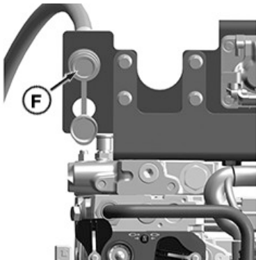
RXA0188466—UN—25JAN23 F—Raccord de carter (vidange du carter moteur)
