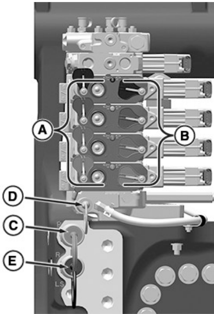
RXA0188465—UN—25JAN23 Débit Standard — Power Beyond dans la pièce moulée d'attelage
