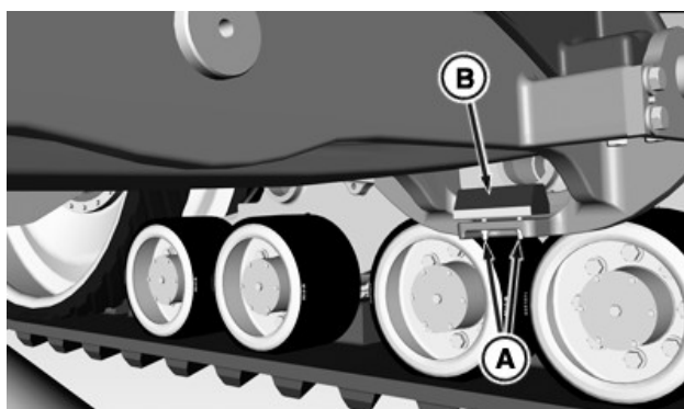
A—Écrou (2) B—Butée inférieure gauche
