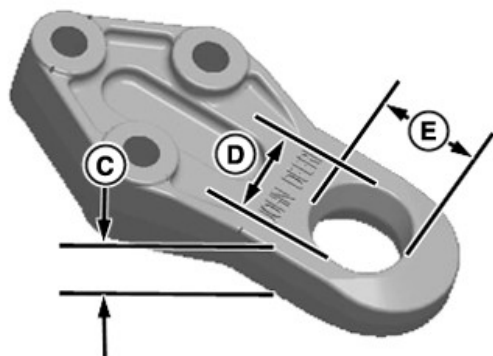
Dimensions de l'articulation du relevage
