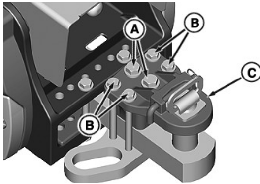
RXA0141899—UN—05JUN14 Barre d'attelage renforcée
