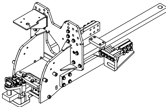
RXA0074740—UN—03MAY04 Support de barre d'attelage renforcé, capacité 4990 kg (11 000 lb)
