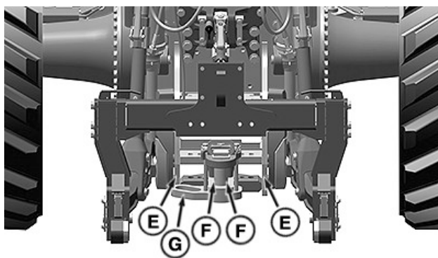
Avec attelage
