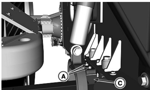
A—Écrou (2) C—Butée supérieure droite
