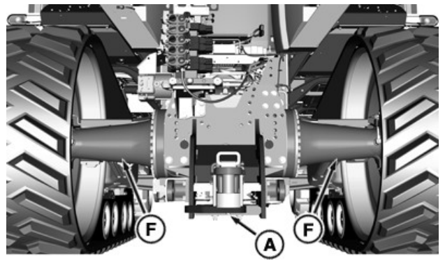
Point de levage arrière
