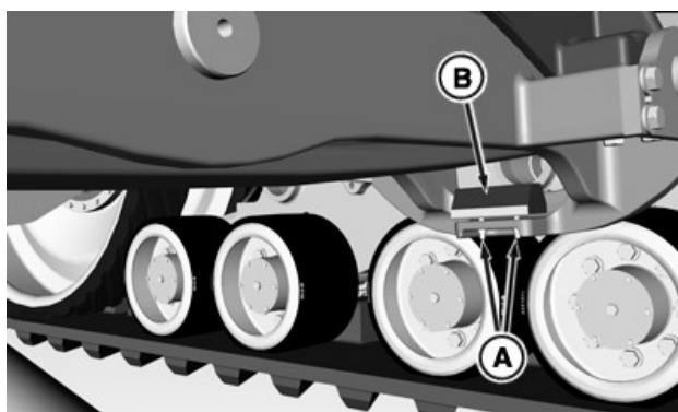
A—Écrou (2) B—Butée inférieure gauche
