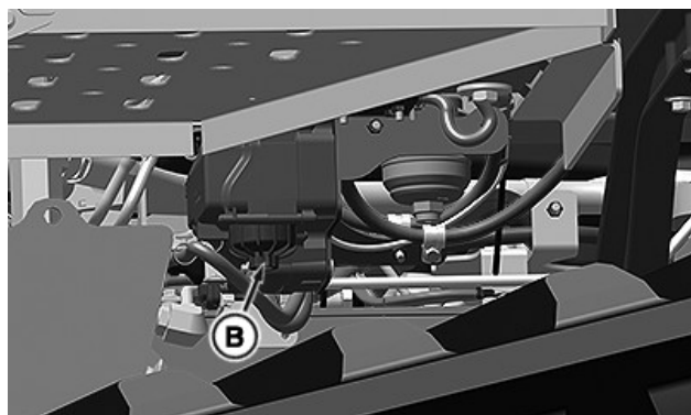
Le filtre du système d'injection d'urée DEF (B) se trouve sous les marches de gauche.
