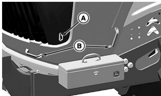
Déverrouillage du capot moteur et poignées du capot moteur
