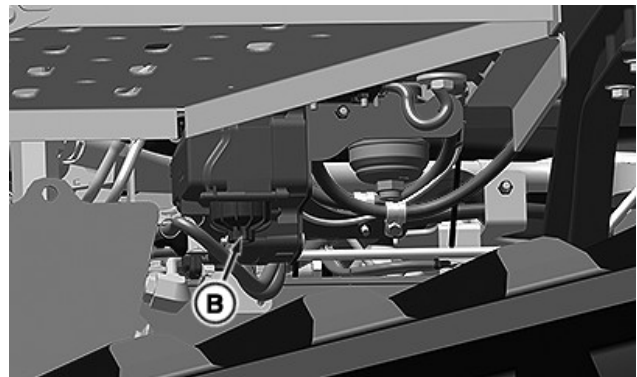
El filtro de la unidad de dosificación de DEF (B) está situado debajo de los peldaños de la izquierda.
