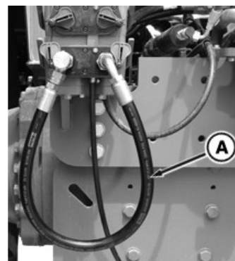
Anschluss des Überbrückungsschlauchs an SCV-Anschlusskupplung [Schürfkübel]
