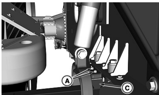
Pufferanschlag rechts oben
