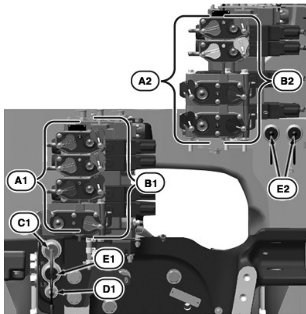
SCV mit hohem Durchfluss mit Anschlusskupplungen I – VIII
