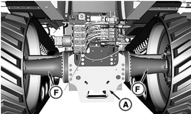
Hinterer Hebeplatz
