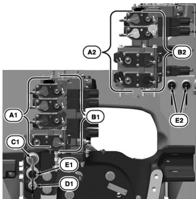
SCV-Block für Hydrauliksystem mit hohem Durchfluss – Acht SCVs mit Zusatzdruckversorgung im Gussteil der Anhängerkupplung
