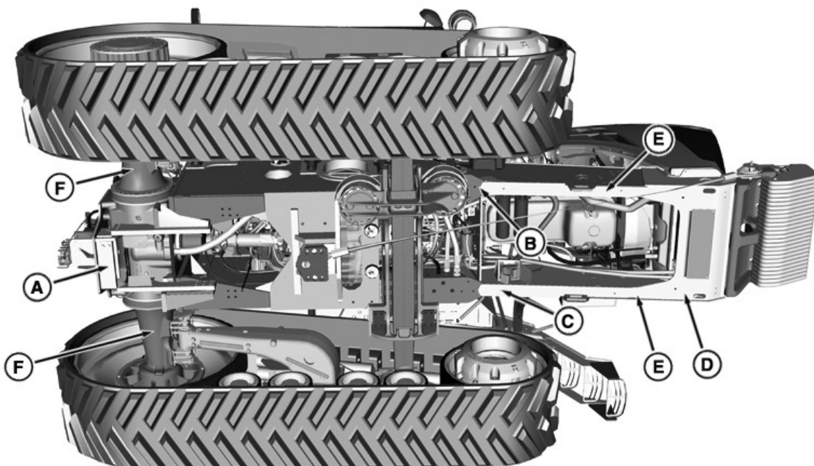
Unterseite, Hebepunkte
