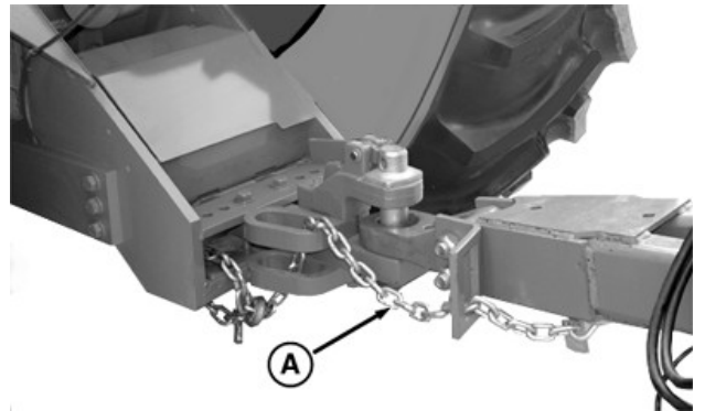
Standard-Zugpendel
