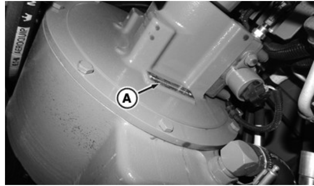
Seriennummer der Zapfwellenkupplung (A) befindet sich hinten an der Zapfwellenkupplung
