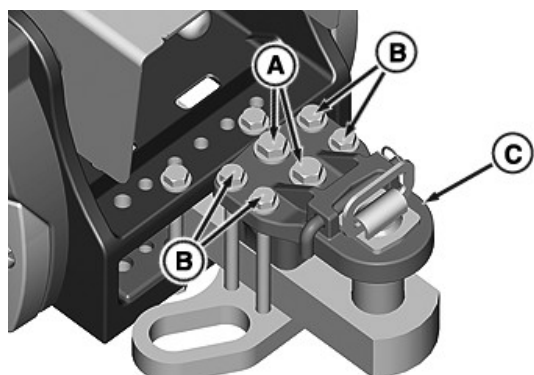
Barre d'attelage renforcée
