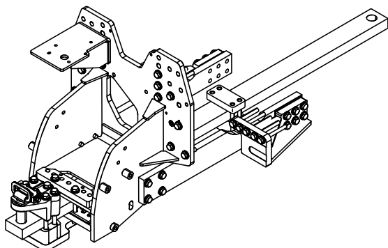
Support de barre d'attelage renforcée, capacité 4990 kg (11000 lb)
