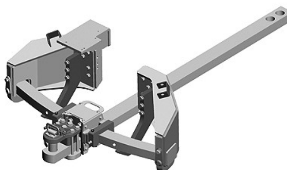
Support de barre d'attelage à grand débattement avec jeu de support à haute capacité, capacité 5440 kg (12000 lb)
