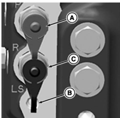
Raccord de bloc de puissance hydraulique externe—Pièce moulée d'attelage
