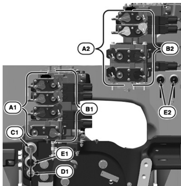
Bloc de distributeurs auxiliaires hydrauliques à haut débit
