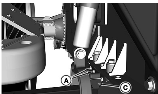
RXA0142144—UN—05JUN14 Butée supérieure droite
