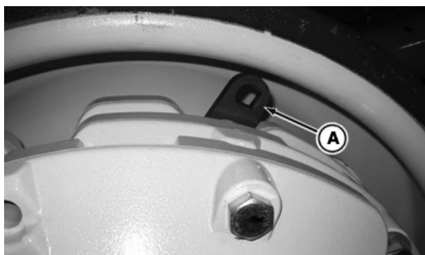
RXA0100328—UN—03FEB09 Clé de maintien pour masse de lestage de roue JDG10958
