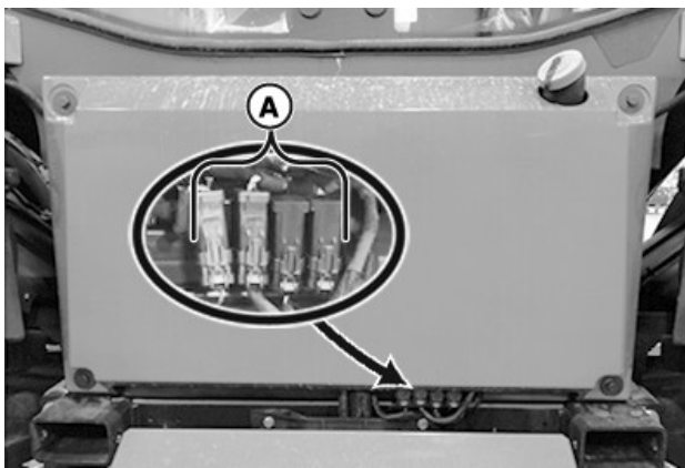
Machine équipée d'un processeur 4600
