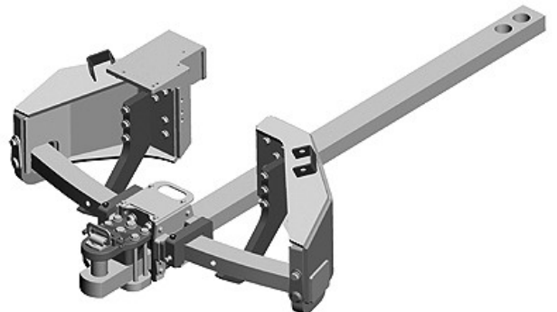
Support de barre d'attelage à grand débattement avec jeu de support à haute capacité, capacité 5440 kg (12000 lb)
