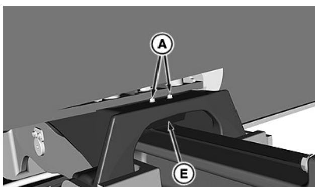
RXA0142146—UN—05JUN14 Butée supérieure gauche
