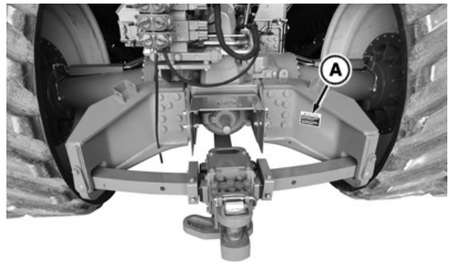
A— Etiqueta de la barra de tiro de giro ancho
