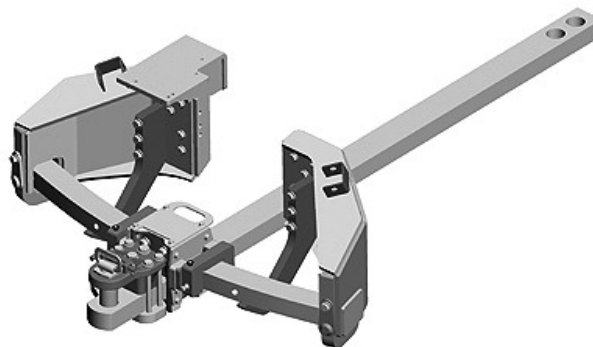
RXA0098007—UN—06MAY08 Soporte de barra de tiro de giro ancho con juego de soporte de alta capacidad, 5440 kg (12000 lb) de capacidad
