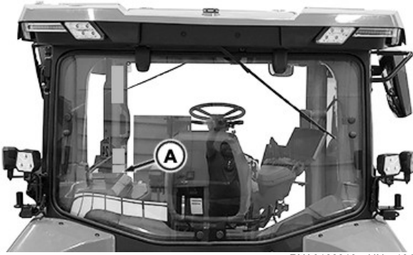
A—Etiqueta de advertencia de transporte, estructura protectora contra vuelcos y cinturón de seguridad
