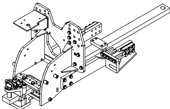
RXA0074740—UN—03MAY04 Soporte de barra de tiro reforzada, 4990 kg (11000 lb) de capacidad
