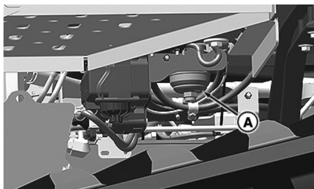
El filtro en línea de fluido de escape diésel (DEF) (A) se encuentra debajo de los escalones izquierdos.
