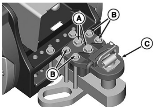
RXA0141899—UN—05JUN14 Barra de tiro reforzada
