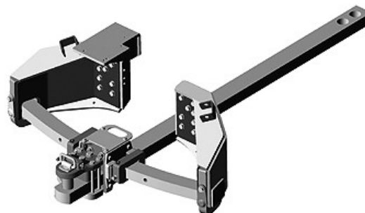
RXA0098006—UN—06MAY08 Soporte de barra de tiro oscilante ancho, 4580 kg (10100 lb) de capacidad
