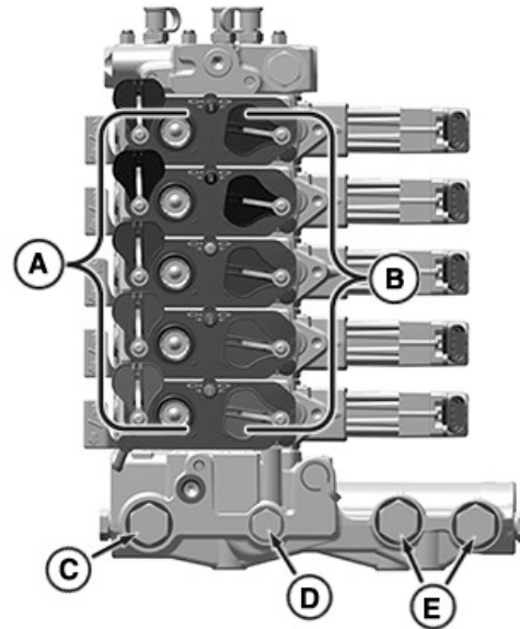
Débit Standard — Power Beyond à l'emplacement supérieur
