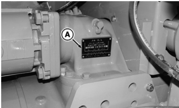
RXA0142510—UN—12JUN14 La chapa de identificación (A) del eje se encuentra en la carcasa del eje trasero
