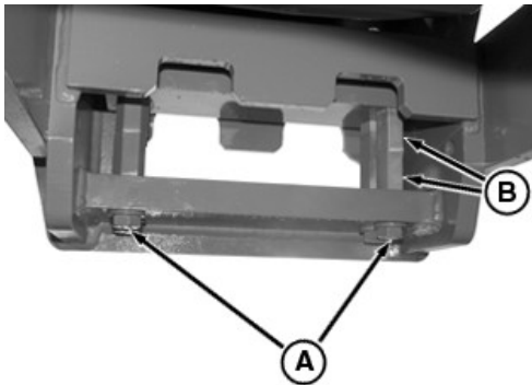
RXA0082010—UN—05JUL05 Instalación del soporte de la barra de tiro más grande de la trailla
