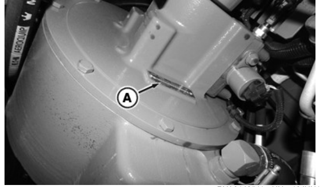
RXA0142511—UN—16JUN14 El número de serie del embrague de TDF (A) se encuentra en la parte trasera del embrague de TDF
