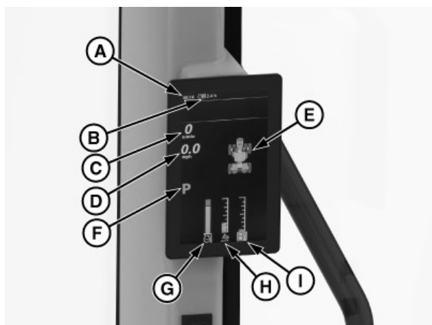
Zaslon na stupu u kutu
