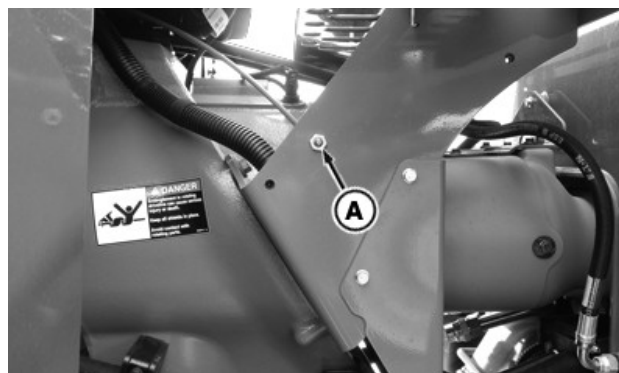
Gornji usadni vijak osovinice šarke
