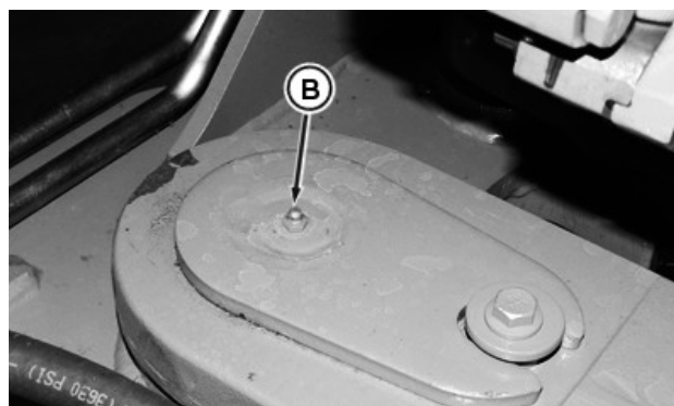
Donji usadni vijak osovinice šarke
