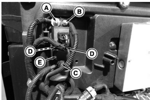
Relaj modula napajanja priključnog uređaja
