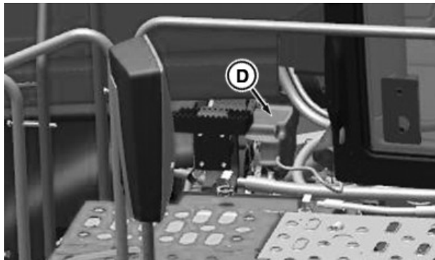
Panel głównych bezpieczników (D) znajduje się po lewej tylnej stronie dolnego wspornika maski.
