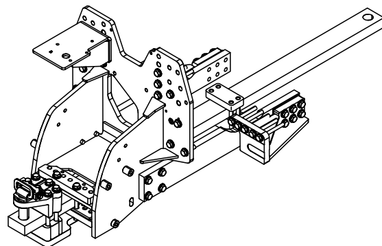
Wspornik wzmacniający do zaczepu rolniczego, udźwąg 4990 kg (11000 lb.)
