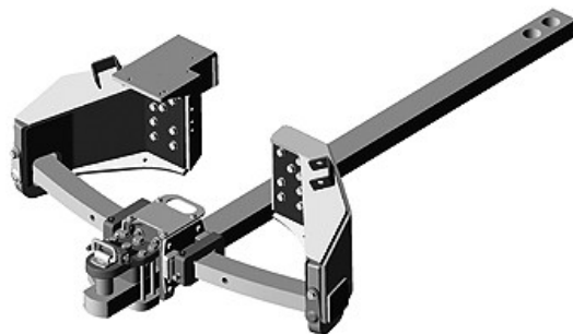
Wspornik zaczepu rolniczego o szerokim promieniu wychylenia, udźwąg 4580 kg (10100 lb.)
