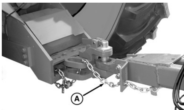
RXA0058318—UN—06NOV01 Standardowy zaczepek rolniczy
