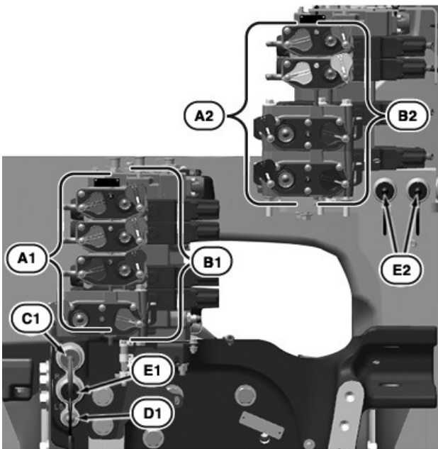
RXA0178746—UN—17NOV20 Blok SCV wysokoprzepływowego układu hydraulicznego — osiem zaworów SCV w przypadku systemu Power Beyond w odlewanym elemencie zaczeput
