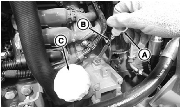
Silnik 13,6 l
