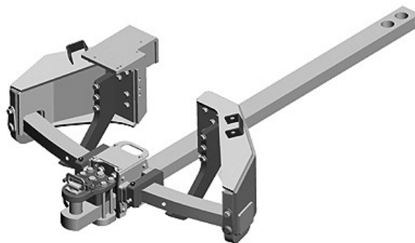
Wspornik zaczepu rolniczego o szerokim promieniu wychylenia z zestawem wspornika wzmocniającego, udźwąg 5440 kg (12000 lb.)
