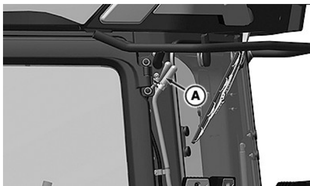
RXA0180428—UN—11NOV20 Filtr odpowietrznika zbiornika DEF (A) znajduje się w górnej części lewego tylnego narożnika kabiny.
