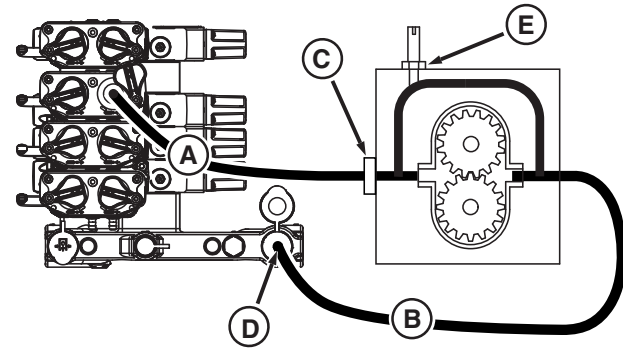
Pompa cieczy opryskowej (bez podnośnika)
