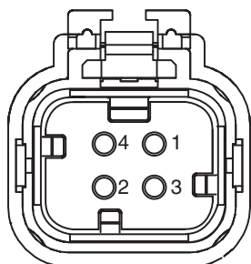
Identyfikacja styku złącza wideo
