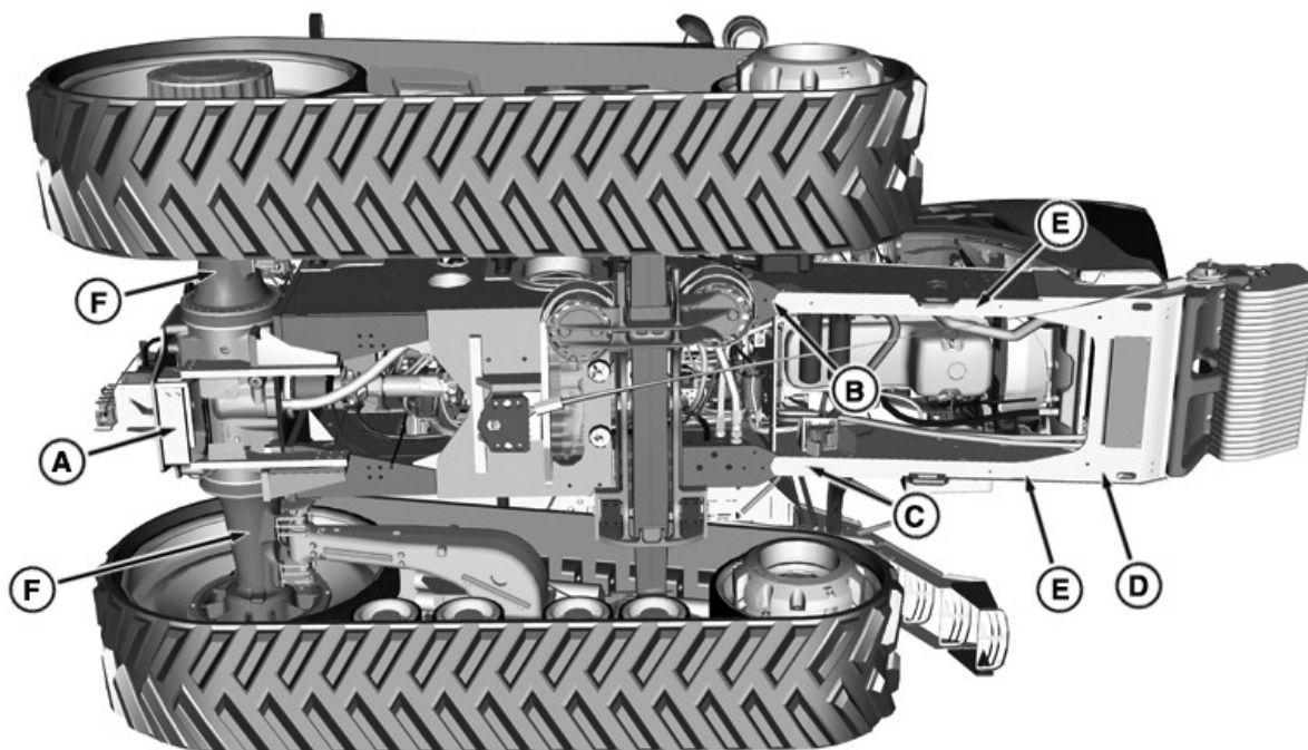
Spodní strana, zvedací místa
