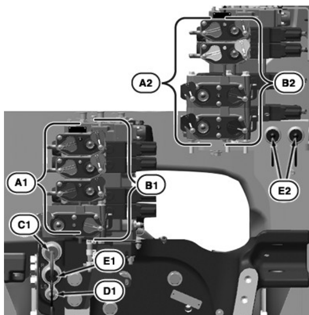
RXA0178746—UN—17NOV20 SCV s vysokým průtokem s přípojkami I–VIII
