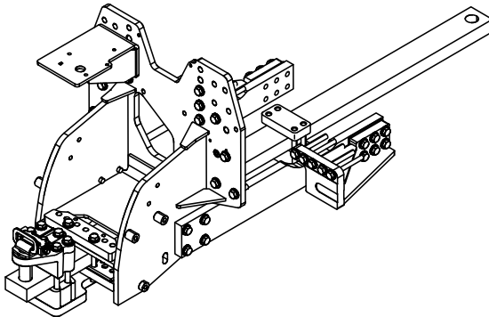
Nagy terhelhetőségű vonórúdtartó 4990 kg (11000 lb) teherbírás
