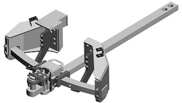
Széles lengő vonórúd támasz, nagy teherbírású támasz készlettel 5440 kg (12000 lb) teherbírás
