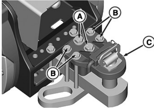
Nagy terhelhetőségű vonórúd
