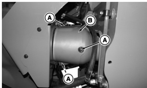
Преграда на задвижващия вал на BOM
