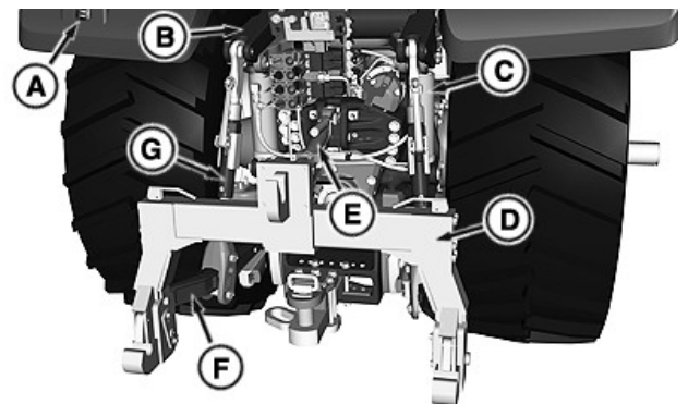
Компоненти на навесната система
