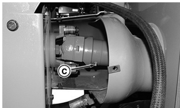
Фитинг на задния силоотводен вал (със свалени части)
