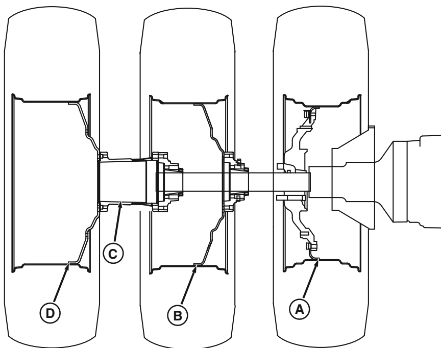
Тройни колела (стандартна главина на колелото)
