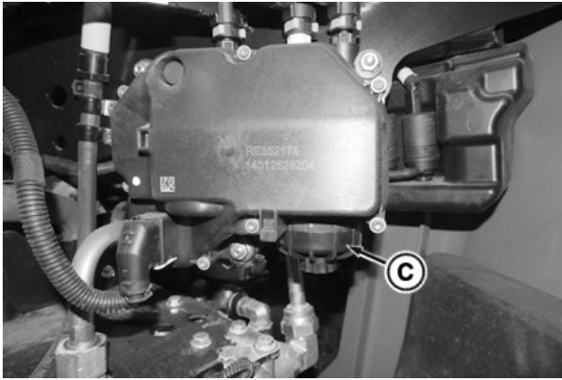
РХА0161214—UN—26ОСТ17 Филтърът (С) на устройството за дозиране на DEF се намира в акумулаторното отделение, на дъното на устройството за дозиране на DEF.
