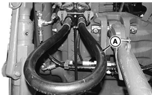
Instalación del manguito auxiliar en el acoplador de la VMD [Ag]
