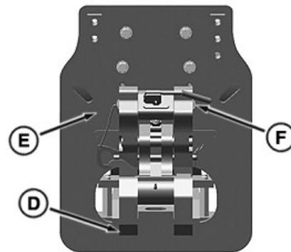
Barra de tiro de acople rápido
