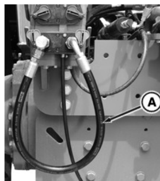
Instalación del manguito auxiliar en el acoplador de la VMD [Trailla]
