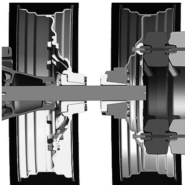
RXA0173134—UN—10DEC19 Imagen 1 del contrapeso de rueda
