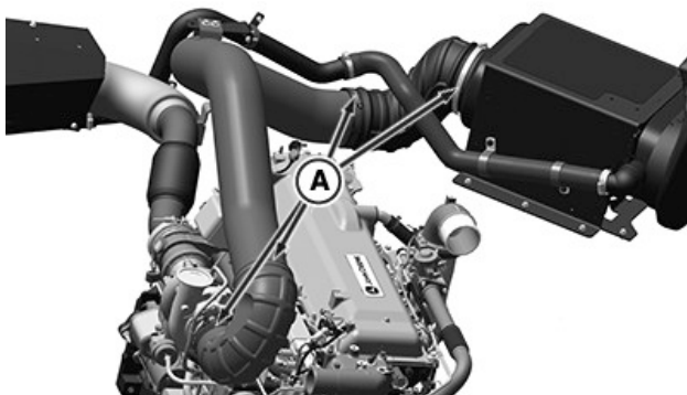
Motor turbo de una etapa
