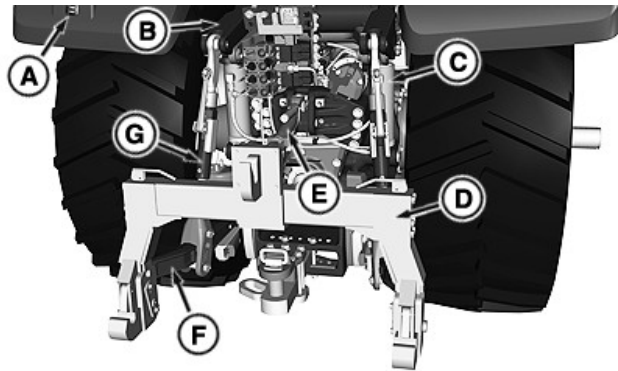
Componenti del sollevatore
