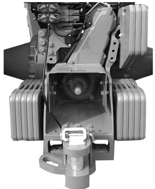
Configurazione di zavorramento massimo con PTO
