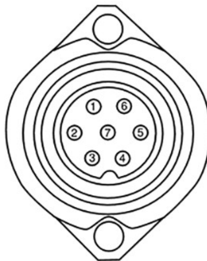
Schema della presa ISO 11786 RXA0169832—UN—05AUG19
