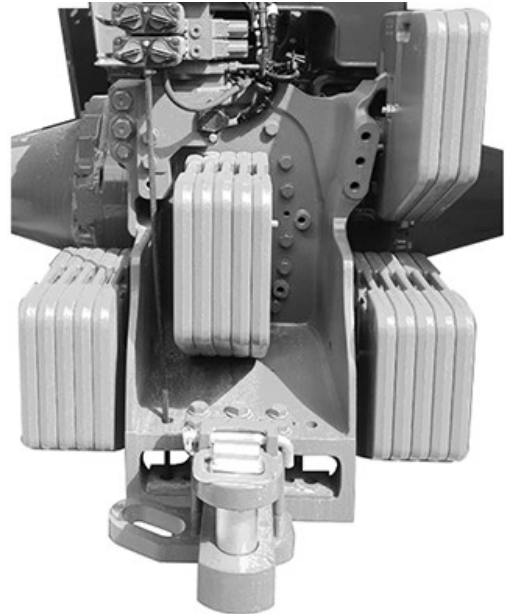
Configurazione di zavorramento massimo senza PTO e sollevatore
