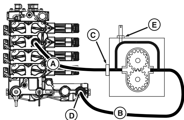
Pompa per l'irrigazione—Senza sollevatore
