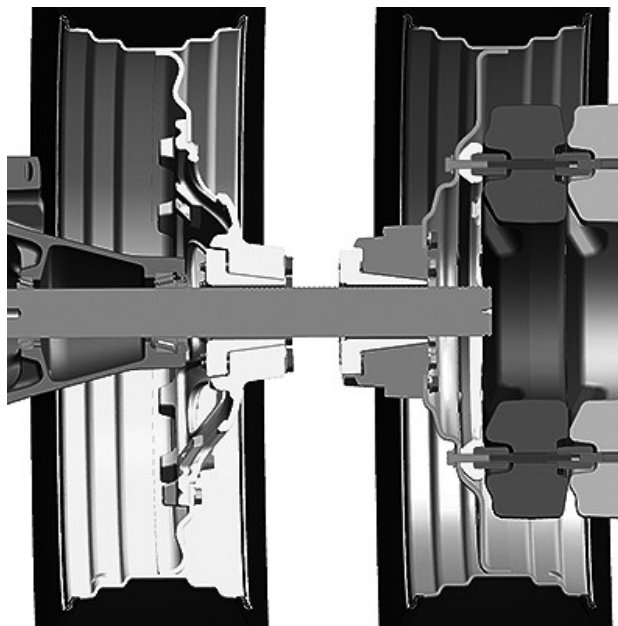
Figura 1 - Peso per ruote
