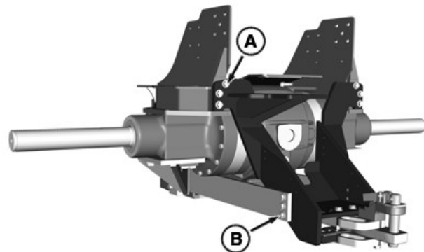
Supporto barra di traino per assale standard a singola riduzione
