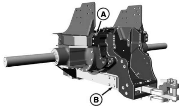
Supporto barra di traino per assale rinforzato a singola riduzione
