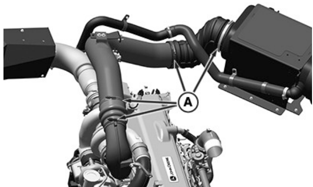
Motor turbo de dos etapas
