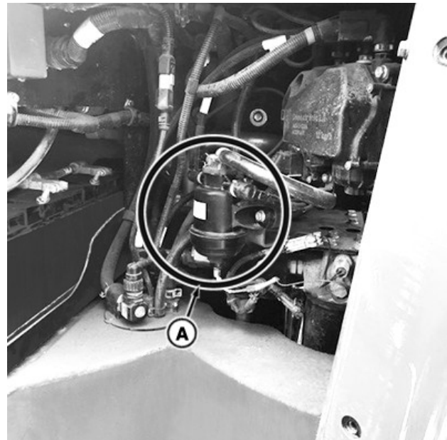
El filtro en línea de fluido de escape diésel (DEF) (A) está dentro del compartimento de la batería.
