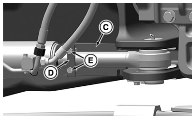
Namontovaný zámok riadenia (ľavá strana)
