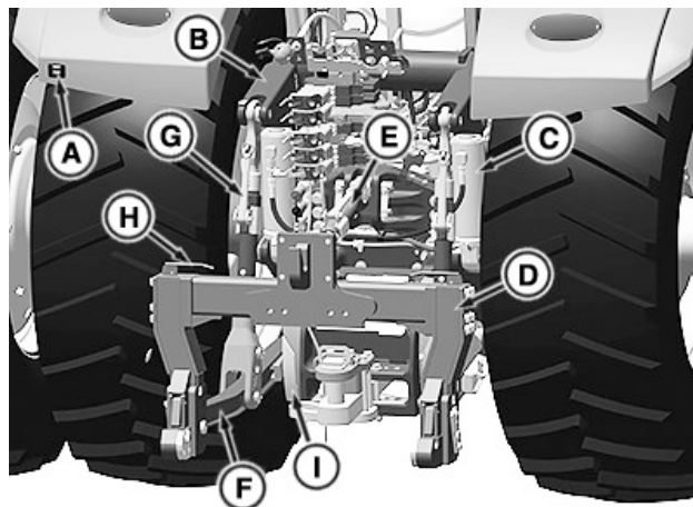
Componentes del enganche trasero
