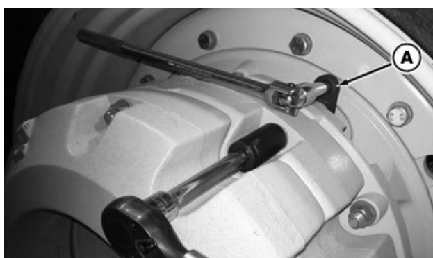
RXA0100329—UN—03FEB09 Závaží vnějšího kola
