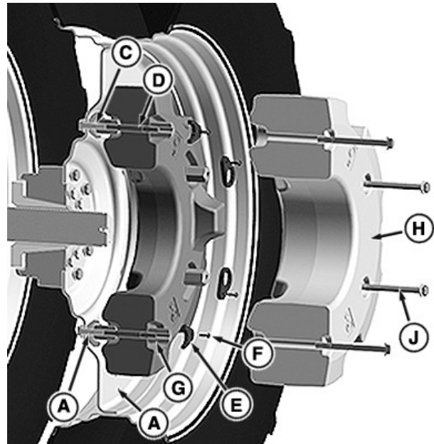
Radgewicht Bild 2
