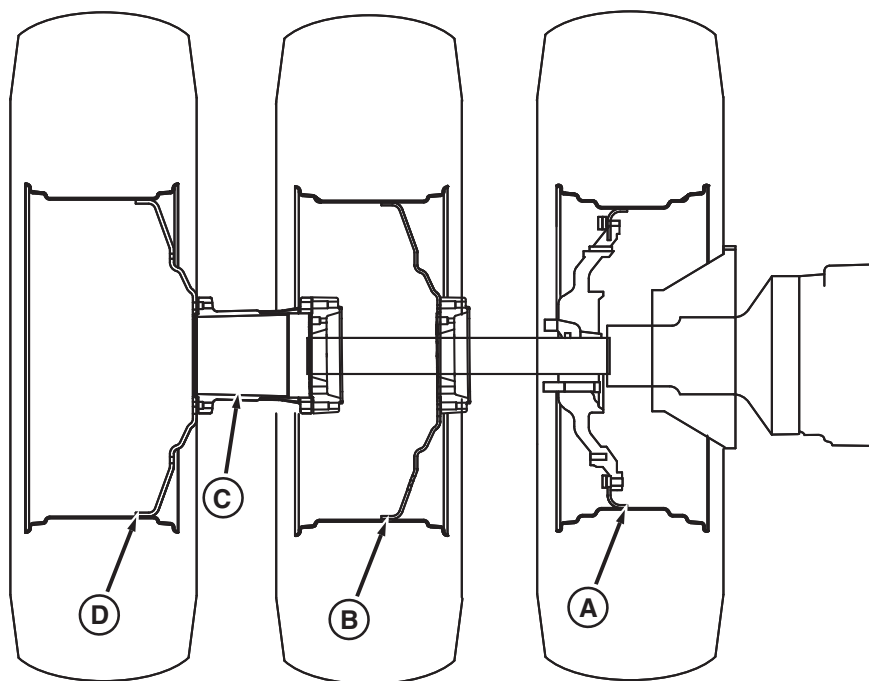
Drillingsräder (Schwerlast-Radnaben)
