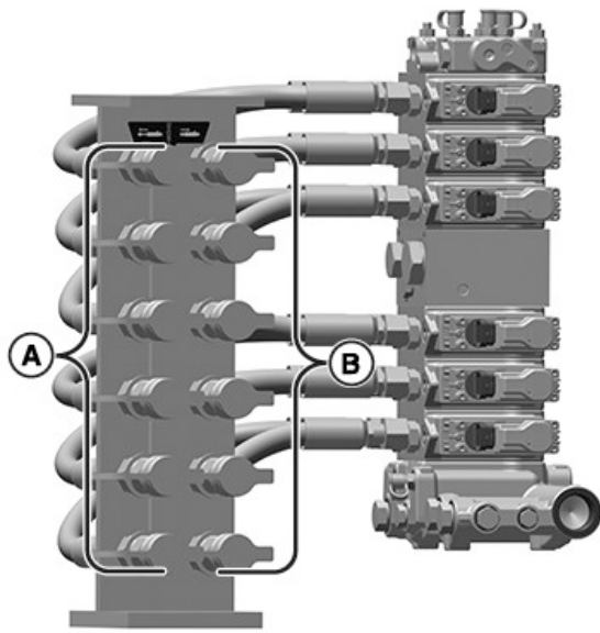
A—Ausfahranschluss (6 St.) B—Einfahranschluss (6 St.)
