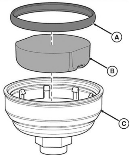
Filtergehäuse – Komponenten
