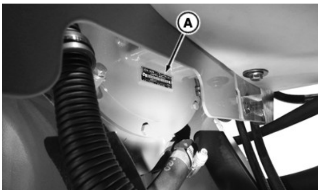
RXA0142514—UN—24JUN14 Jõuvõtuvõlli siduri seerianumber (A) asub jõuvõtuvõlli siduril, pöördetapi lähedal
