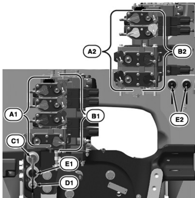
Suure voolukiirusega hüdroväljavõtte liitmikega I–VIII
