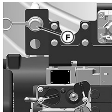
Komponentide tuvastamine ja asukoht [Ag] – suure vooluhulgaga hüdraulika. (F) Õlivanni liitmik – mootori karteri tühjendus
