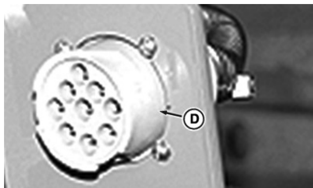
Traktori juhtmekimbu konnektor (D) asub hüdroväljavõtete plokist paremal pool asuva klambri küljes
