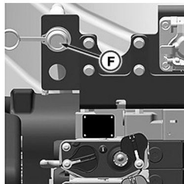
Komponentide tuvastamine ja asukoht [Ag] – suure vooluhulgaga hüdraulika. (F) Ölivanni liitmik – mootori karteri tühjendus
