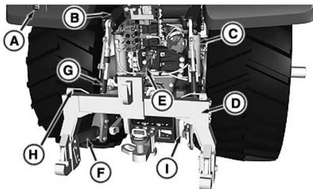
Tagumise haakeseadise komponendid
