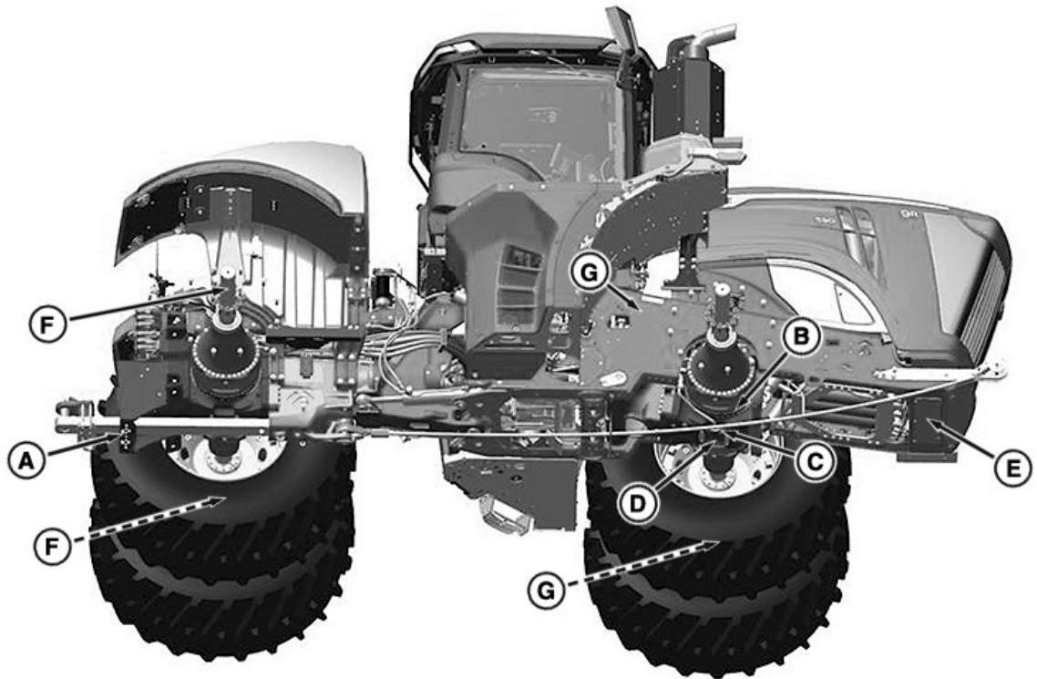
Alumine pool, tõstepunktid
