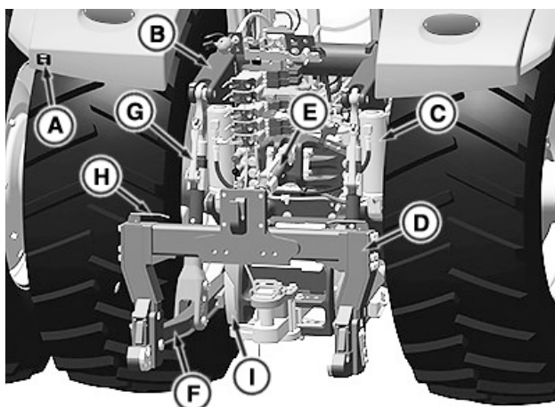
RXA0188513—UN—06FEB23 Компоненты задней навески
