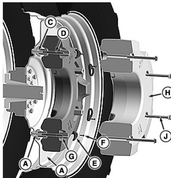
Колісна противага, зображення 2
