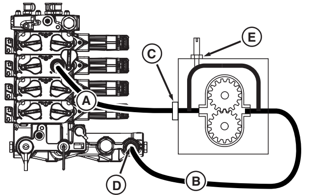
RXA0188469—UN—25JAN23 Спринклерний насос (без зчіпки)
