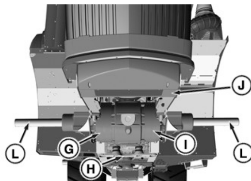
Передні точки підйому (спереду)
