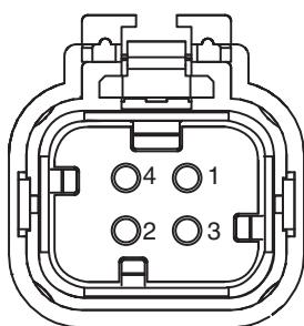
Идентификација на пин за приклучокот за видео
