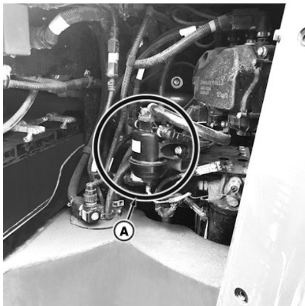
RXA0163952—UN—24JUL18 Линискиот DEF филтер (A) е во преградата за акумулаторот.
