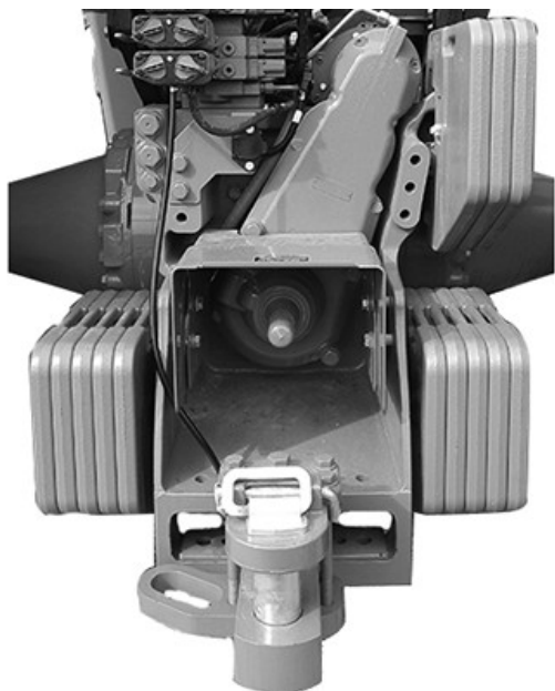
RXA0153814—UN—07SEP16 Конфигурација со максимален баласт со PTO
