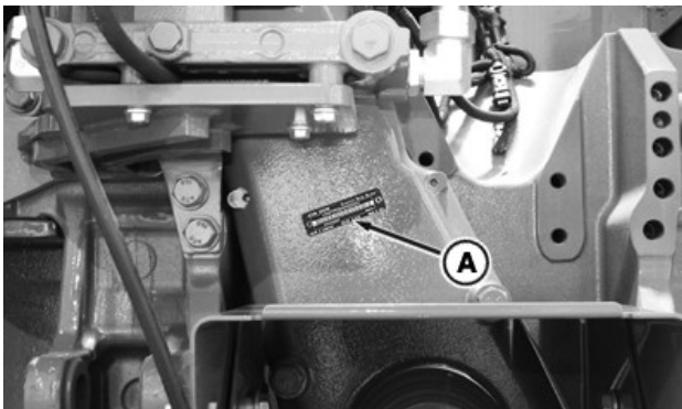
Серискиот број на куќиштето на преносниот механизам на РТО (А) се наоѓа куќиштето на преносниот механизам на РТО на задната страна на тракторот
