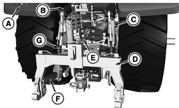
Haakeseadme komponendid
