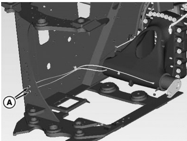
Esisilla vedrustuse tagumiste pukside joonis
