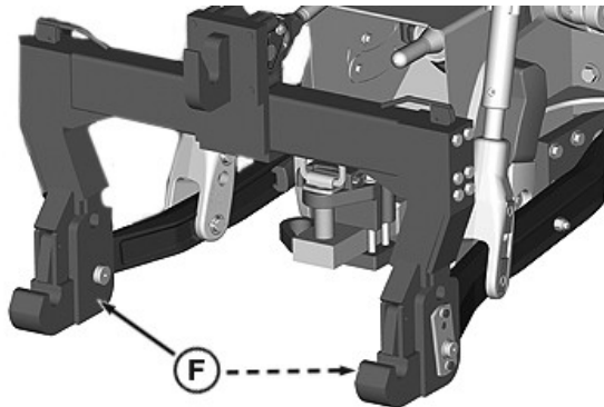
RXA0184147—UN—22JUN21 Näidatud on kiirhaakur kategooria 4N konfiguratsioonis
