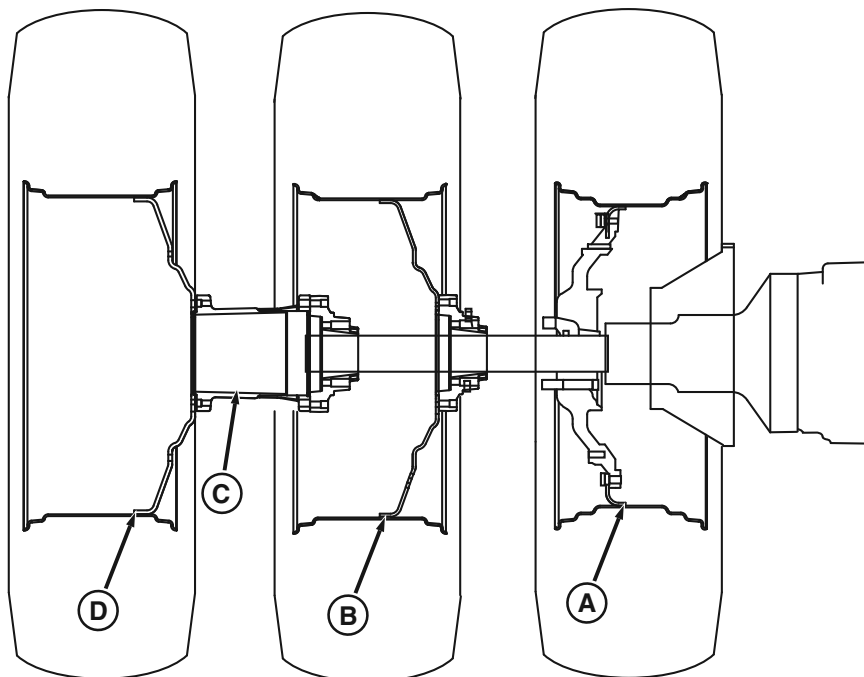
Kolmikrattad (standardrummud)
