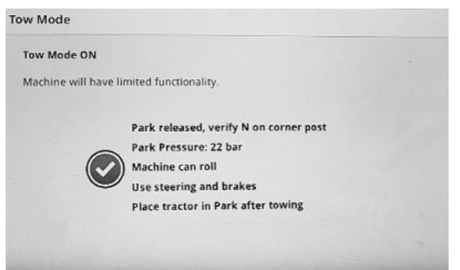
Pukseerimisrežiimi parkimisrõhk
