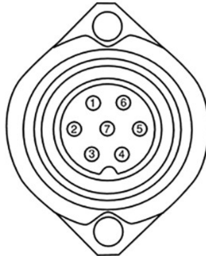
RXA0169832—UN—05AUG19 Schéma de la prise ISO 11786
