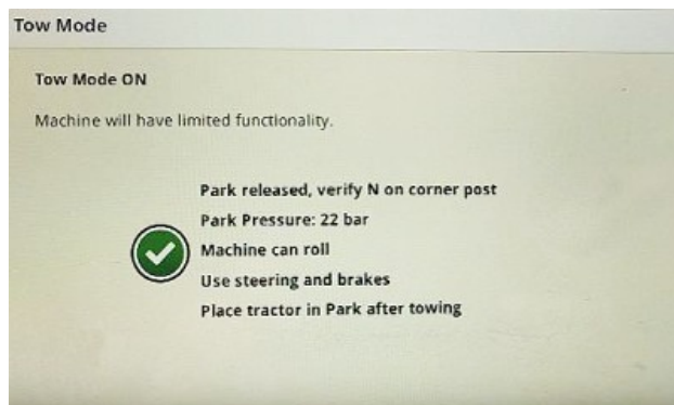
RXA0190401—UN—30JUL24 Pression de stationnement en mode remorquage
