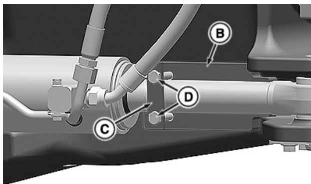
RXA0188672—UN—23FEB23 Namontovaný zámok riadenia (ľavá strana)
