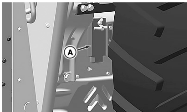
RXA0188670—UN—23FEB23 Zámok riadenia uložený (ľavá strana)
