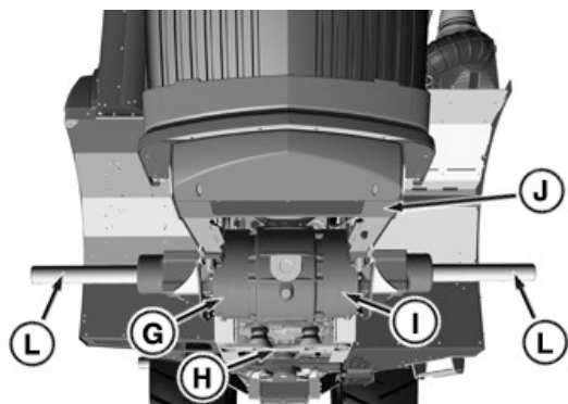
RXA0188398—UN—20DEC22 Zdvíhacie body (vpredu)
