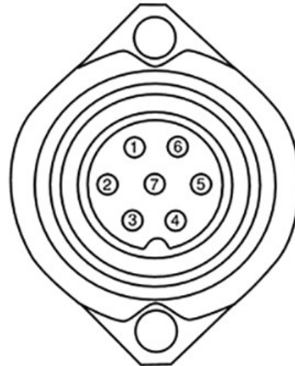
RXA0169832—UN—05AUG19 Schéma zásuvky ISO 11786
